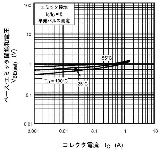
図 7.4 V_{BE(sat)} - I_C
