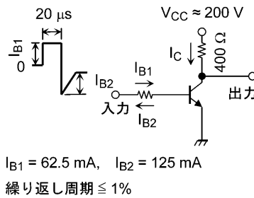
図 5.2.1 スイッチング時間の測定回路
