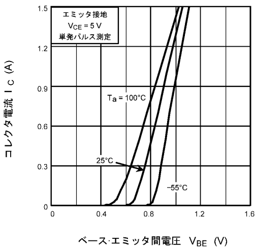
図 7.5 I_C - V_{BE}
