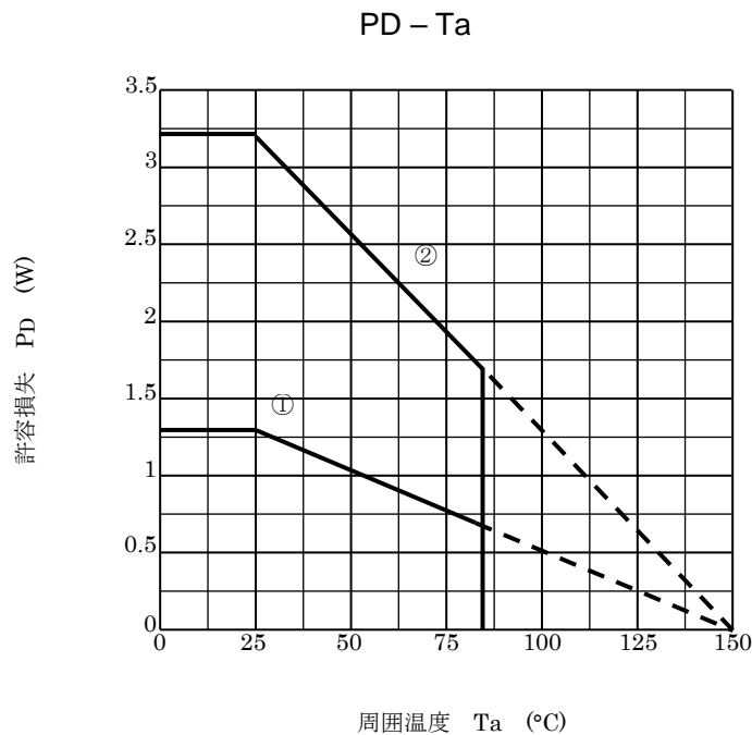
図 10.1 許容損失
