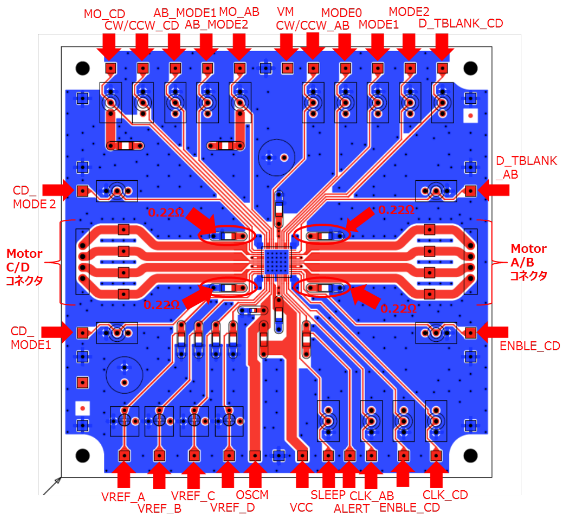
図 11.2 入力関連/主要部品関連 (FTG: QFN48)
