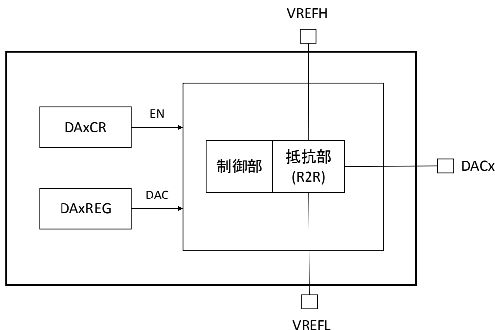
図 2.1 8ビットデジタル/アナログコンバータ ブロック図
