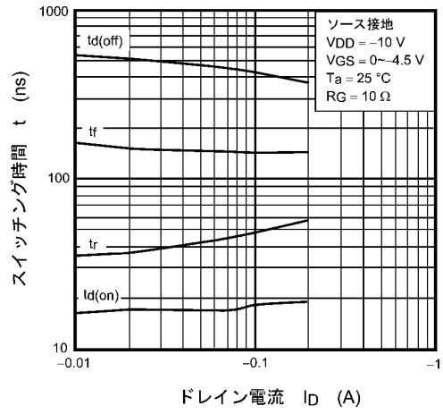
図 7.10 t - I_D
