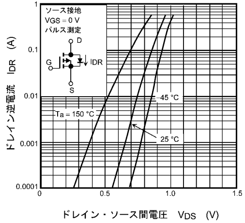
図 7.8 I_{DR} - V_{DS}
