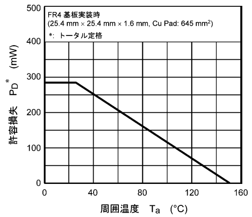
図 7.12 P_D - T_a
