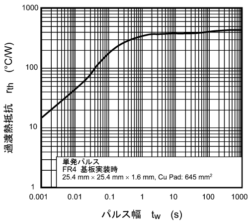
図 8.11 r_{th} - t_w
