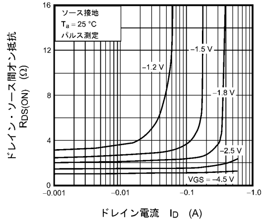
図 7.6 RDS(ON) - ID
