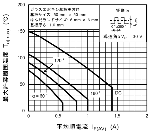
図 10.5 T_{a(max)} - I_{F(AV)}
