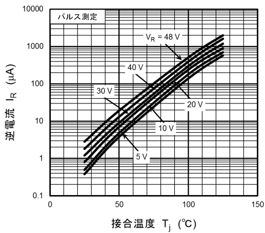
図 10.9 I_R - T_j
