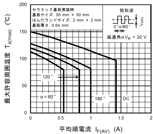
図 10.4 T_{a(max)} - I_{F(AV)}
