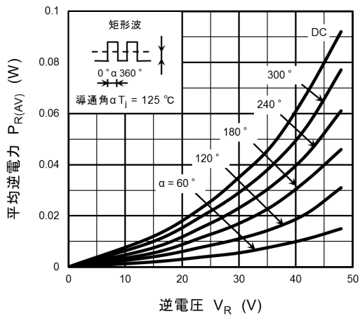
図 10.3 P_{R(AV)} - V_R
