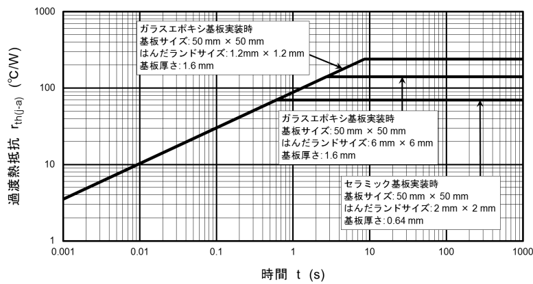
図 10.10 r_{th(j-a)} - t
