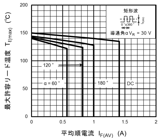
図 10.6 T_{l(max)} - I_{F(AV)}
