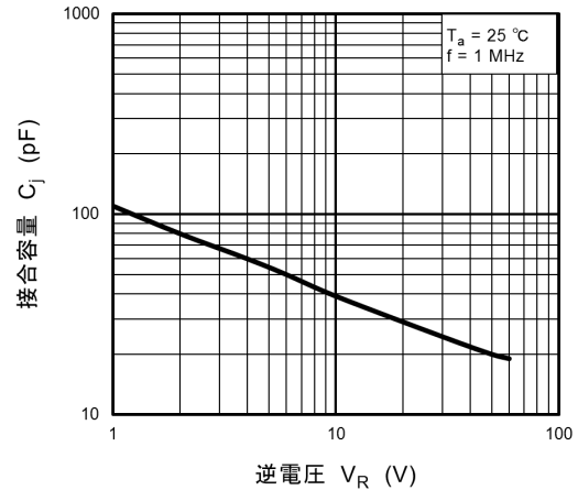
図 10.8 C_j - V_R
