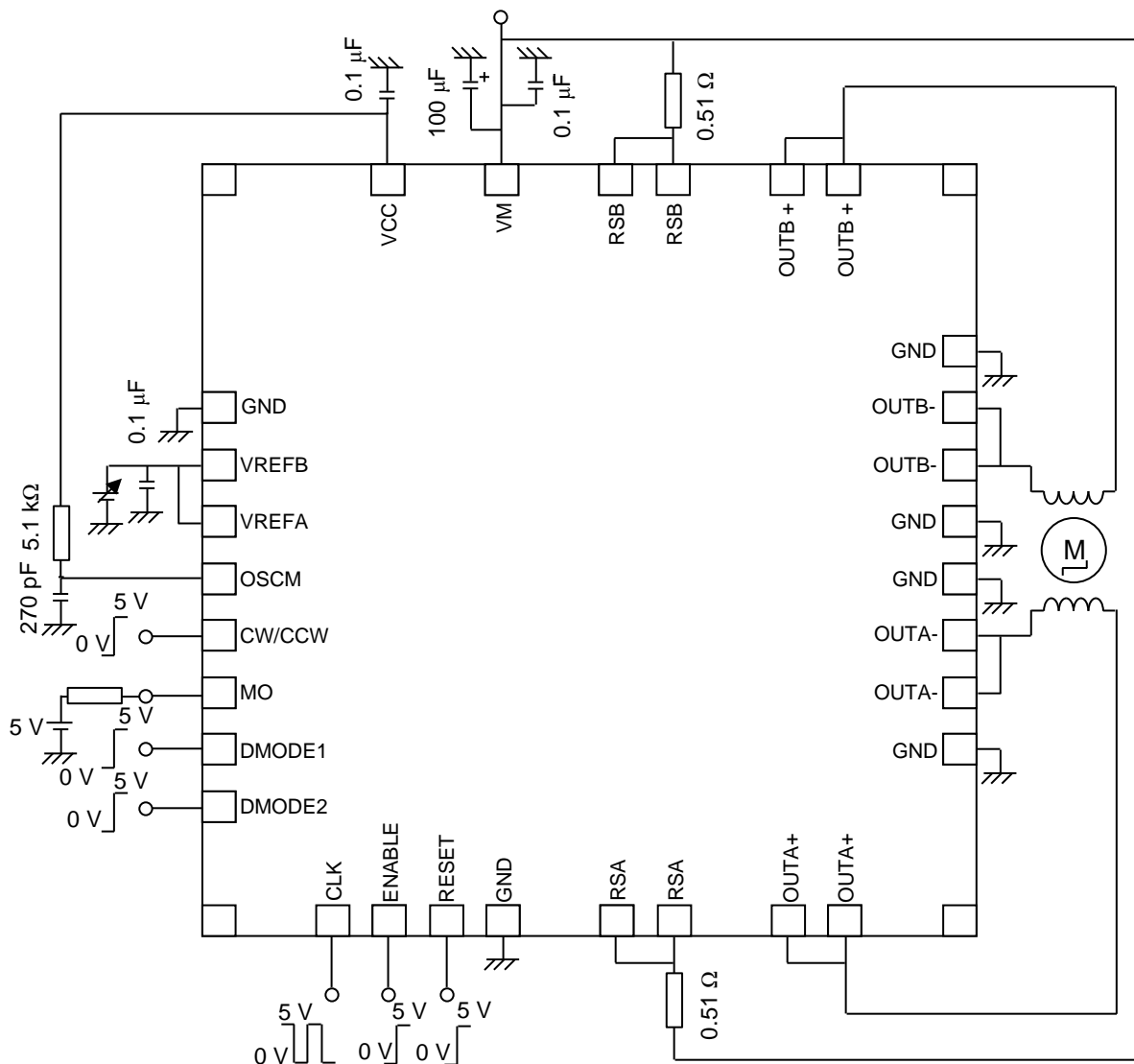
図 10.1 推奨応用回路
