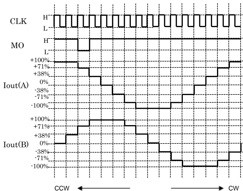
図 6.3 W1-2 相励磁設定
