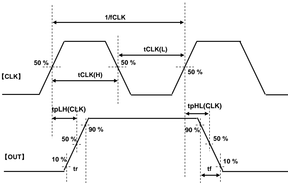
図 9.1 AC 特性タイミングチャート
