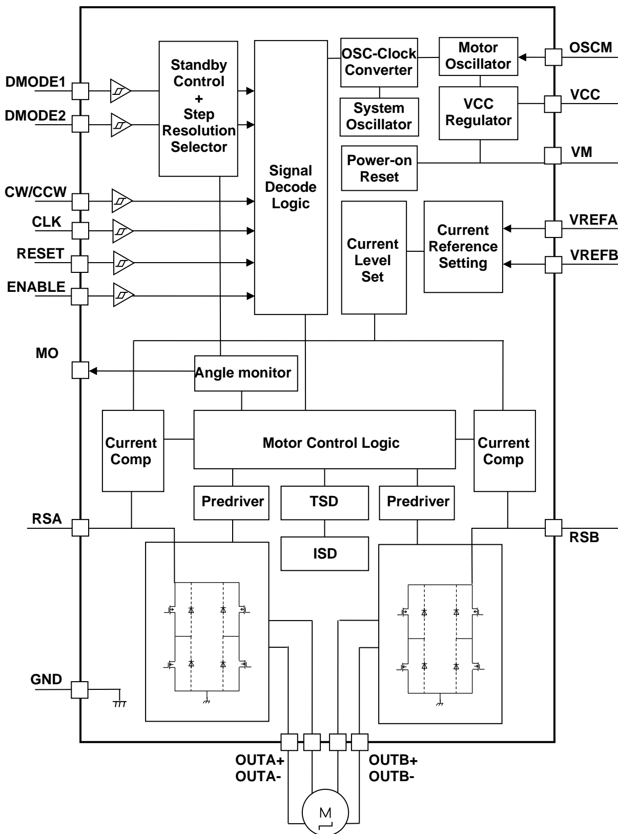
図 3.1 ブロック図
