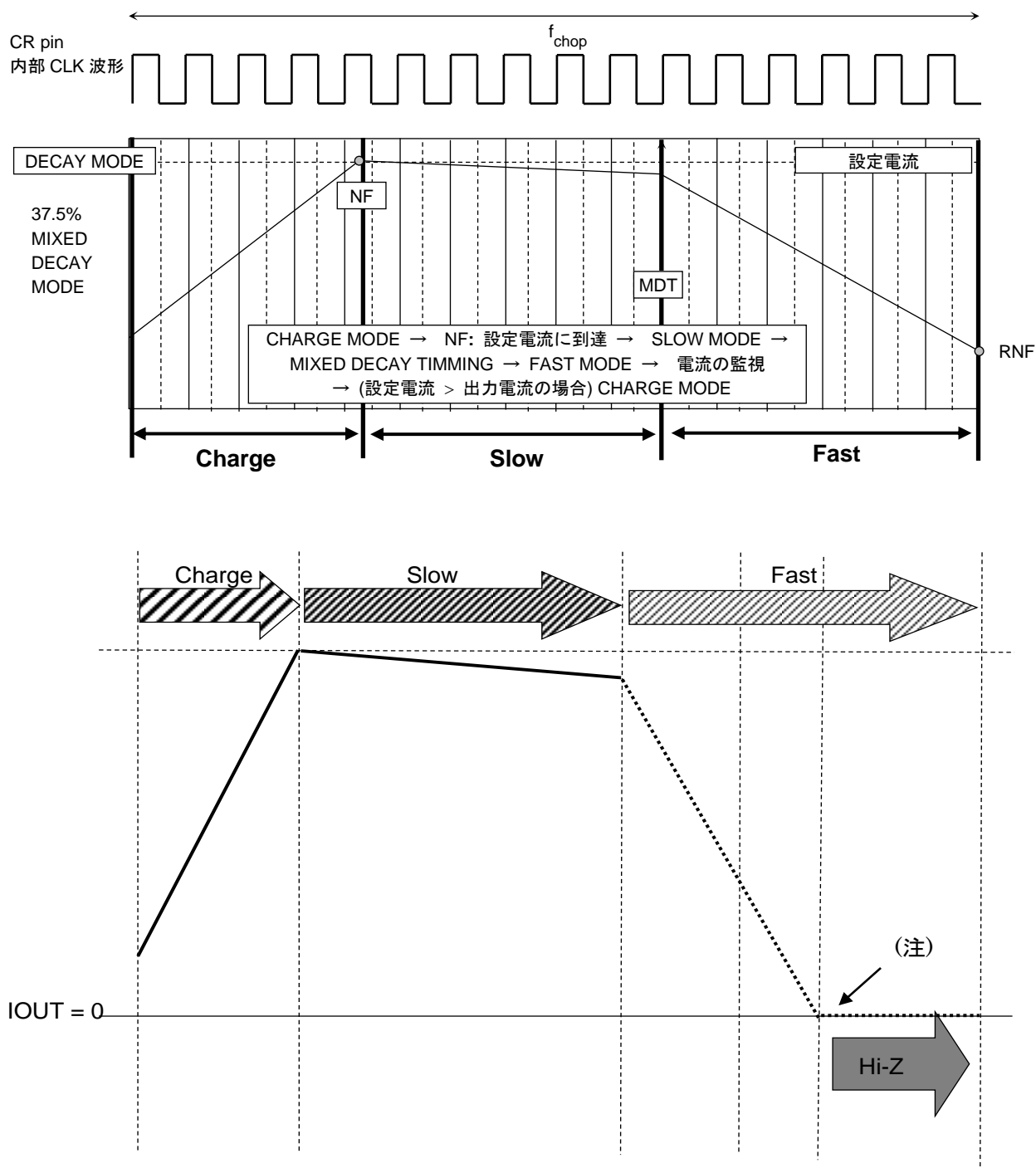
図 6.4 Mixed Decay Mode / 零点検出動作
