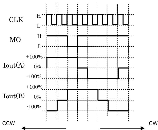
図 6.2 1-2 相励磁設定
