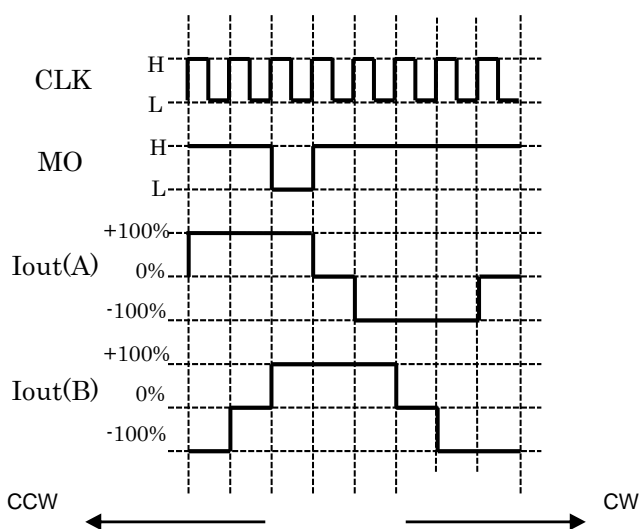
図 6.2 1-2 相励磁設定
