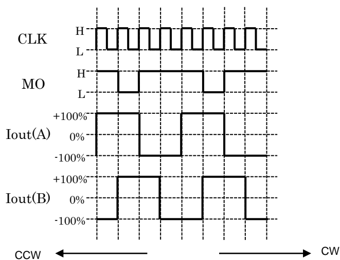
図 6.1 2 相励磁設定
