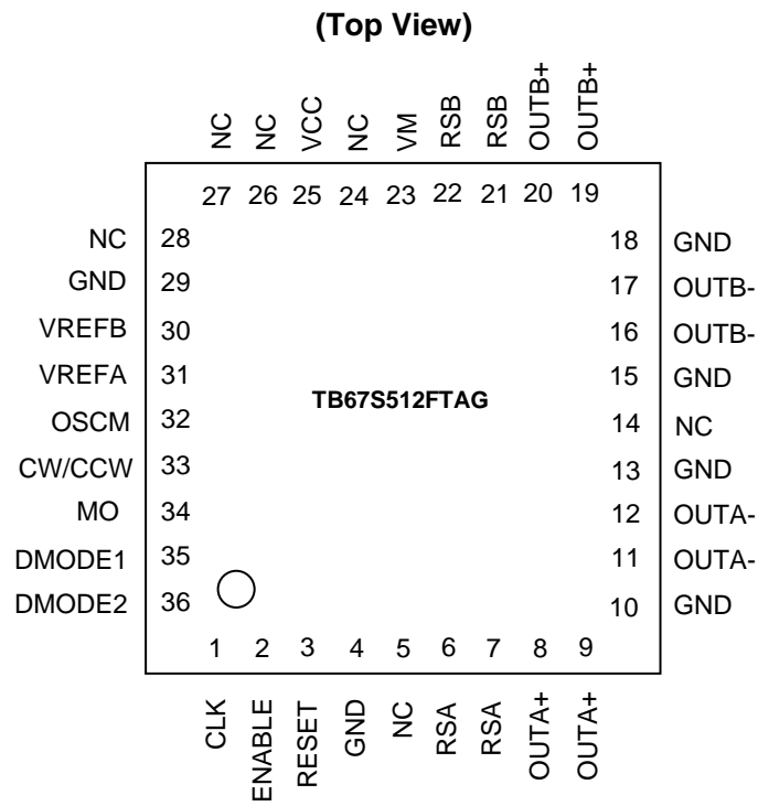
图 4.1 端子配置图
