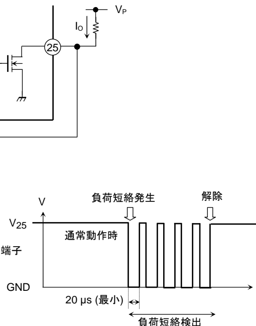
図 10 負荷短絡時 25 ピン出力波形
