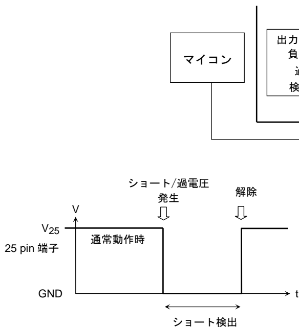
図 9 25 ピン出力波形
