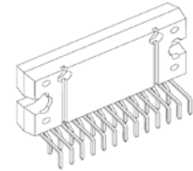
HZIP25-P-1.00F 質量 7.6 g (標準)
