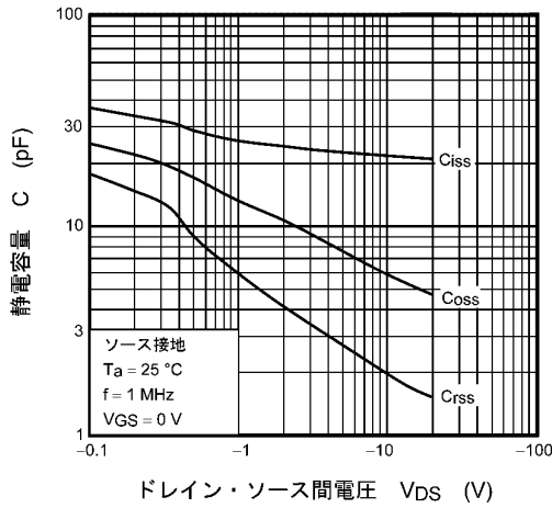
図 7.9 C - V_{DS}
