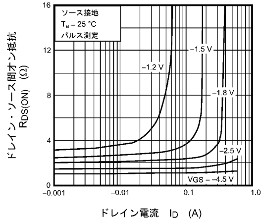
図 7.6 R_{DS(ON)} - I_D
