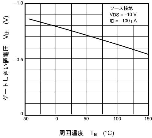
図 7.7 V_{th} - T_a
