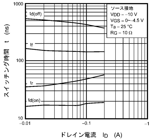
図 7.10 t - I_D
