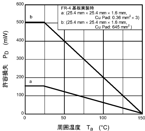
図 7.11 P_D - T_a
