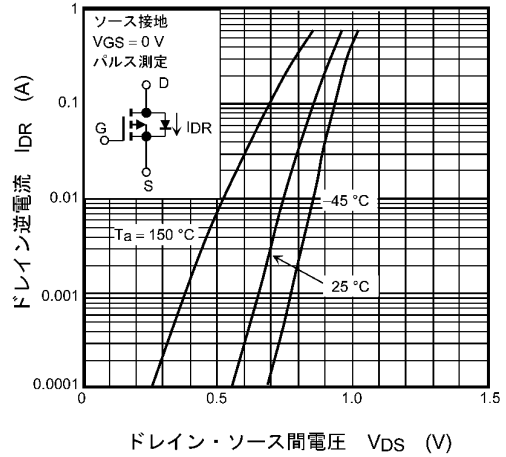
図 7.8 I_{DR} - V_{DS}
