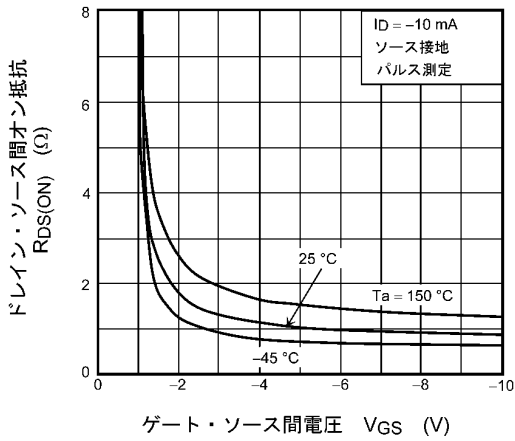
図 7.3 R_{DS(ON)} - V_{GS}
