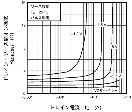
図 7.6 R_{DS(ON)} - I_D
