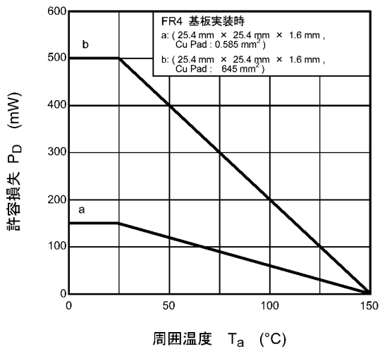
図 8.11 P_D - T_a
