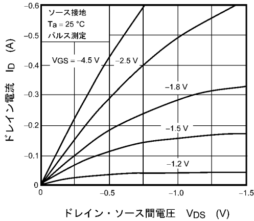
図 7.1 I_D - V_{DS}
