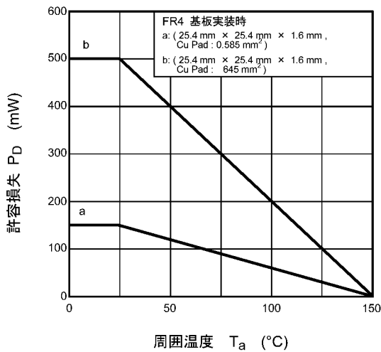
図 7.11 P_D - T_a
