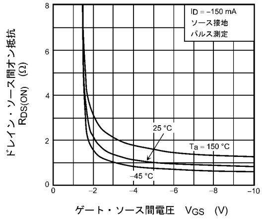
図 7.4 R_{DS(ON)} - V_{GS}
