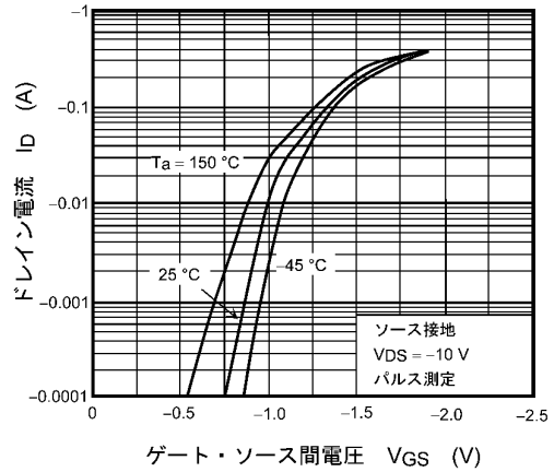
図 7.2 I_D - V_{GS}
