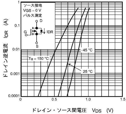
図 8.8 I_{DR} - V_{DS}
