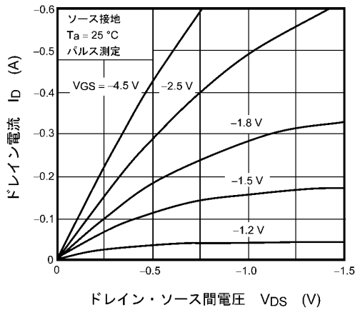
図 7.1 I_D - V_{DS}
