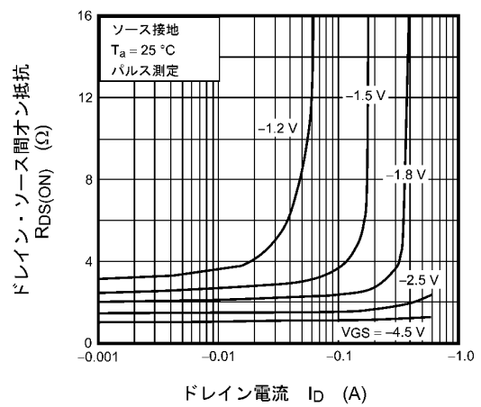
図 7.6 R_{DS(ON)} - I_D
