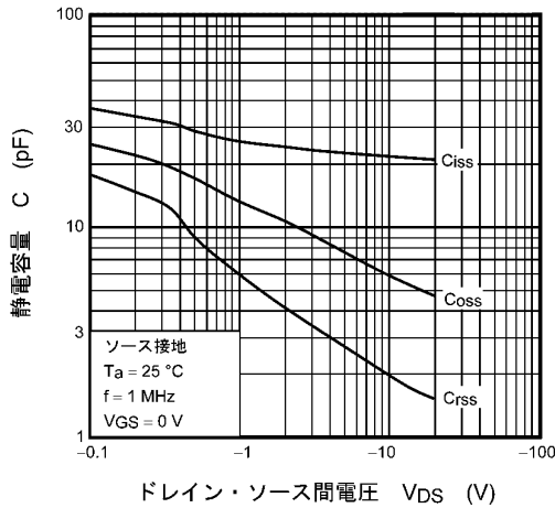
図 8.9 C - V_{DS}
