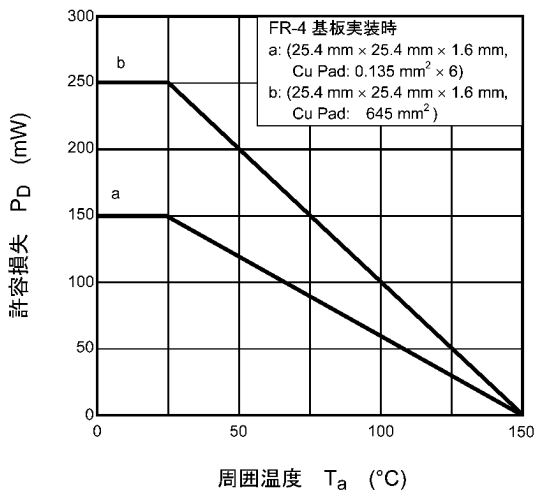
図 7.11 P_D - T_a
