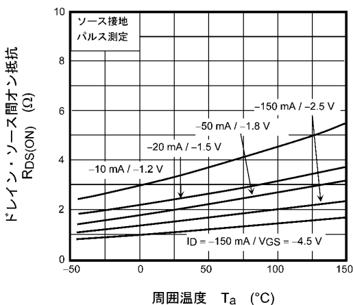
図 7.5 R_{DS(ON)} - T_a
