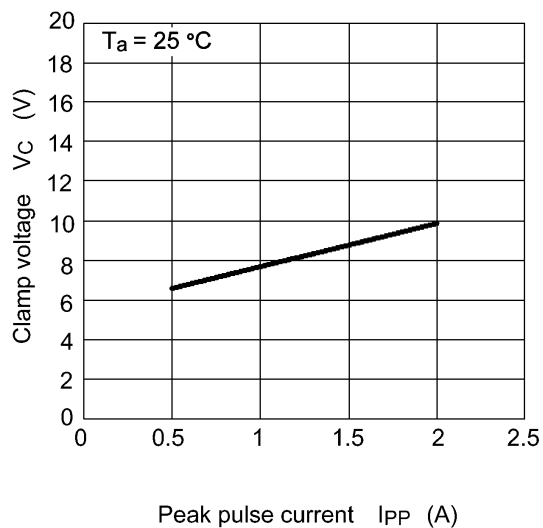
図 6.3.1 V_C - I_{PP}
