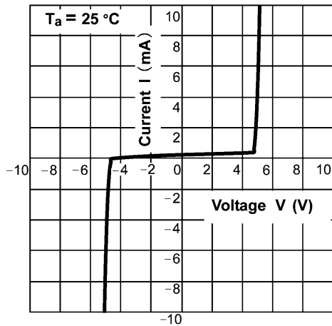
図 9.1 I - V
