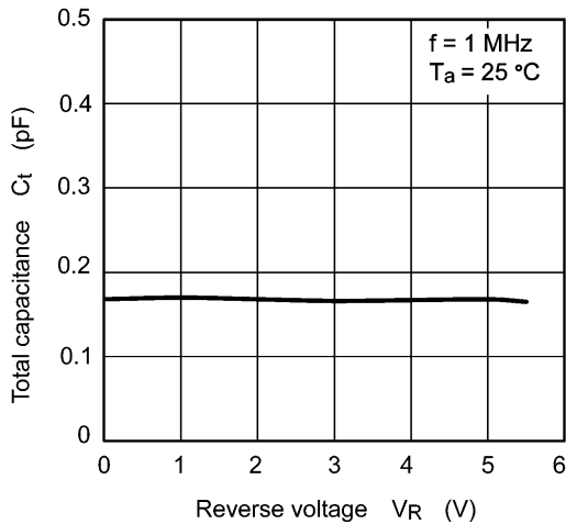
図 9.3 C_t - V_R
