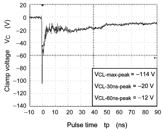
図 6.1.2 -8 kV
