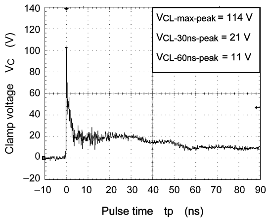
図 6.1.1 +8 kV
