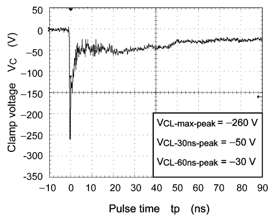
図 6.1.4 -15 kV
