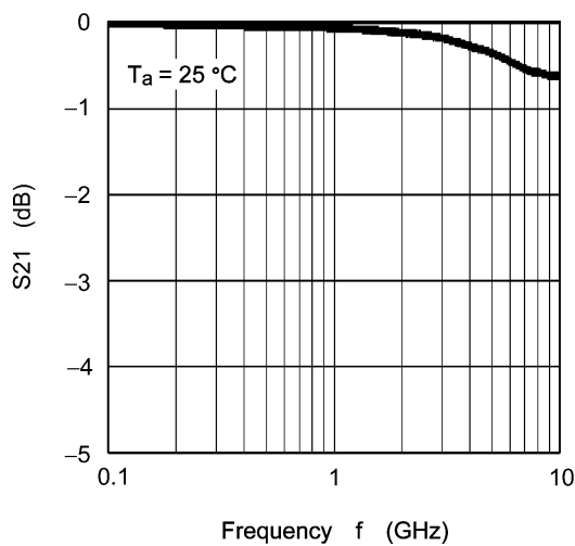
図 9.5 S_{21} - f
