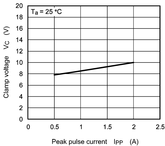
図 6.3.1 V_C - I_{PP}
