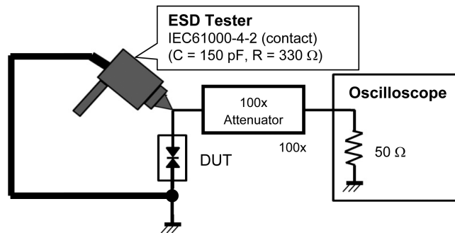
Fig. 6.1.5 IEC61000-4-2 (Contact)
