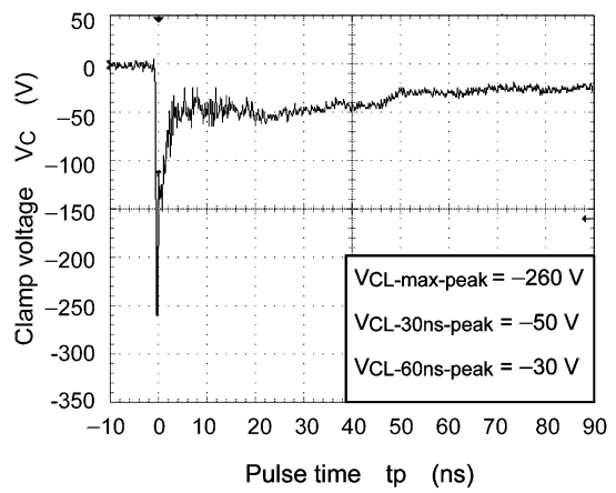
Fig. 6.1.4 -15 kV
