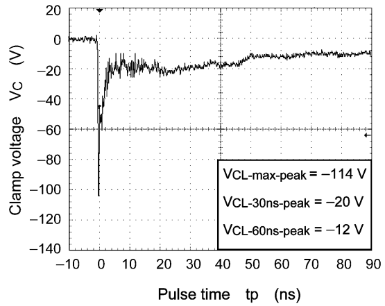
Fig. 6.1.2 -8 kV
