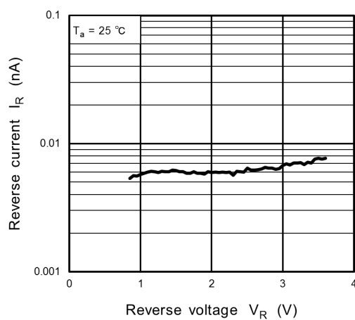
Fig. 9.2 I_R - V_R
