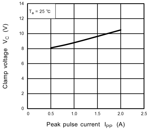
Fig. 6.2.1 V_C - I_{PP}
