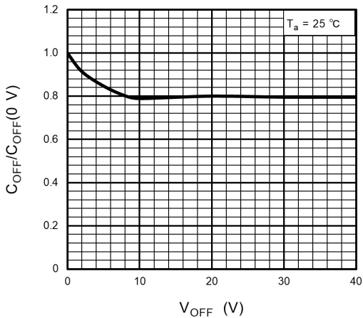
Fig. 14.1.11 C_{OFF} - V_{OFF}
