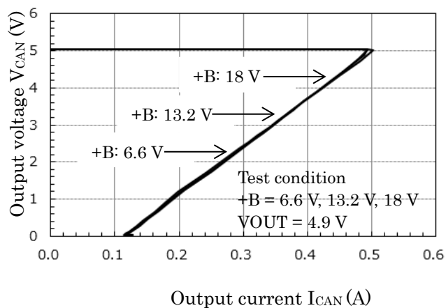
V_{CAN} - I_{CAN}
