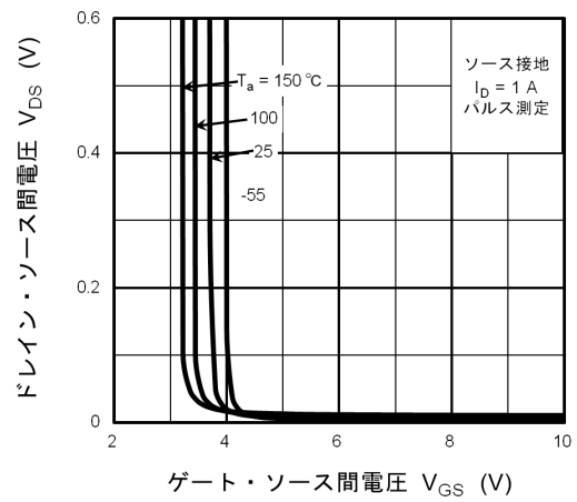
図 9.6 V_{DS} - V_{GS}
