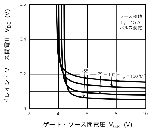
図 9.4 V_{DS} - V_{GS}
