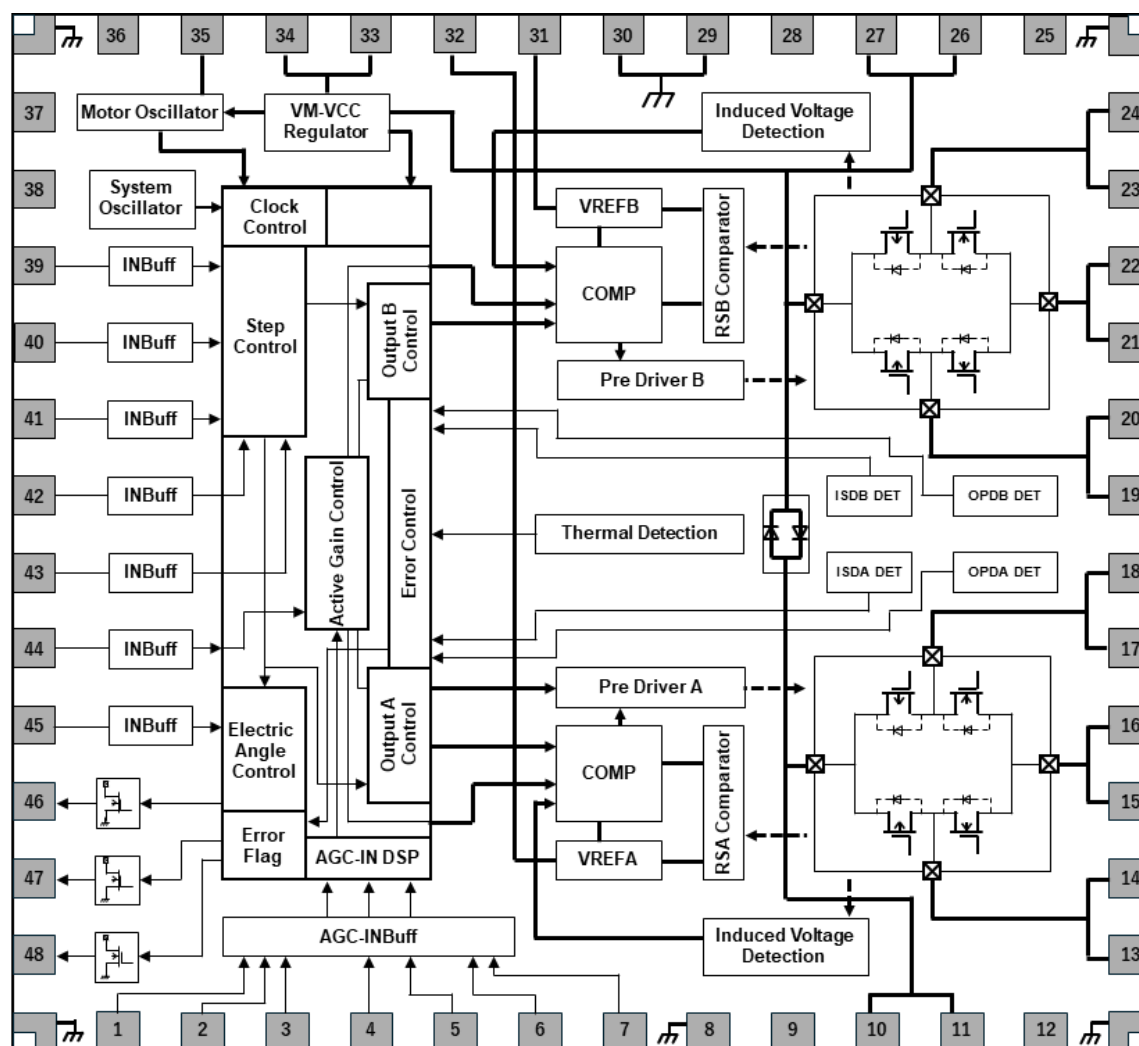
図 5.1 ブロック図
