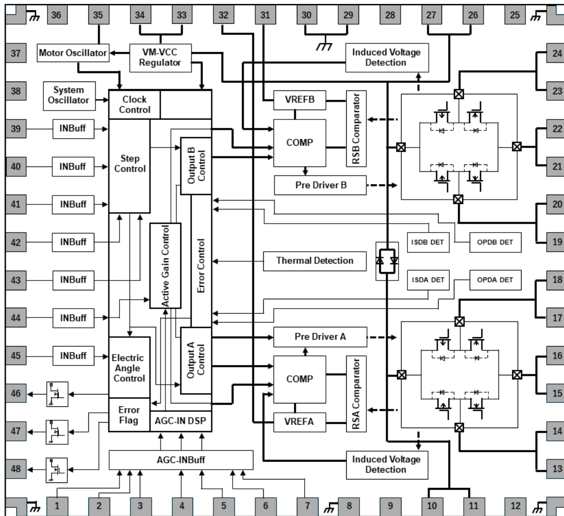
図 5.1 ブロック図
