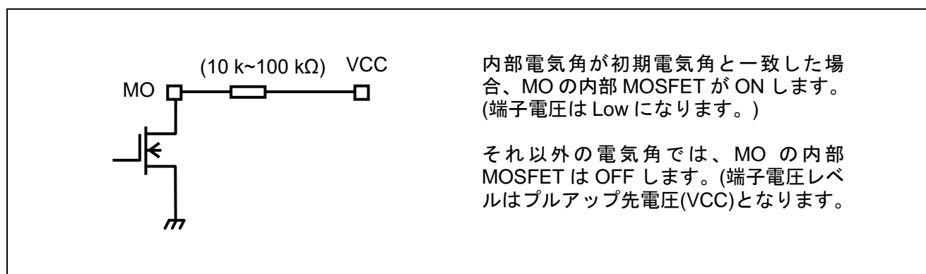
図 7.1 MO ファンクション等価回路
