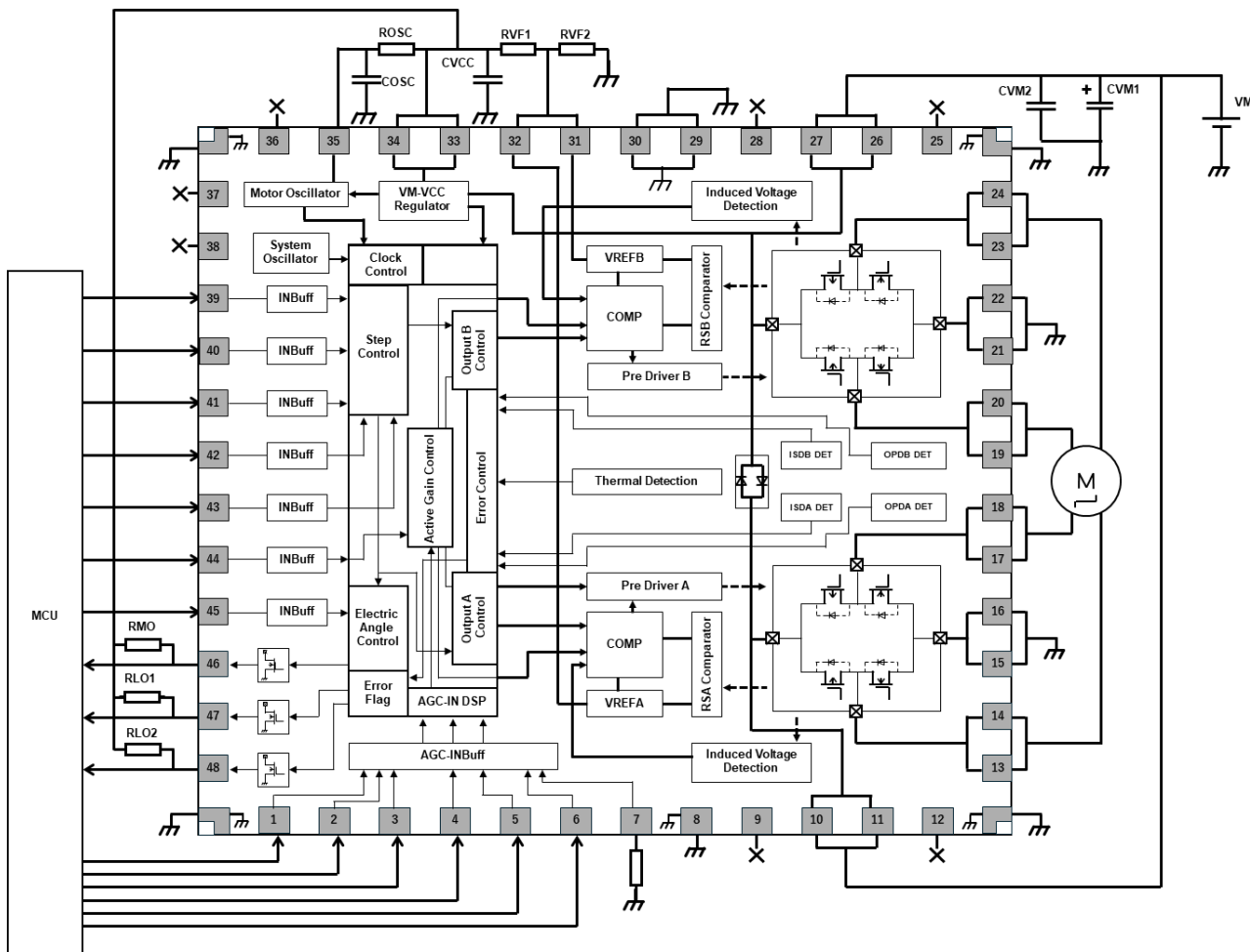
図 11.1 応用回路例
