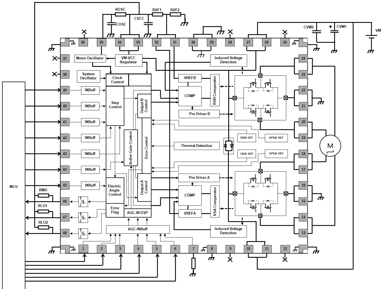
図 11.1 応用回路例
