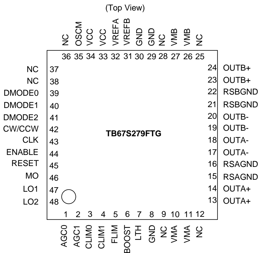
図 3.1 端子配置図
