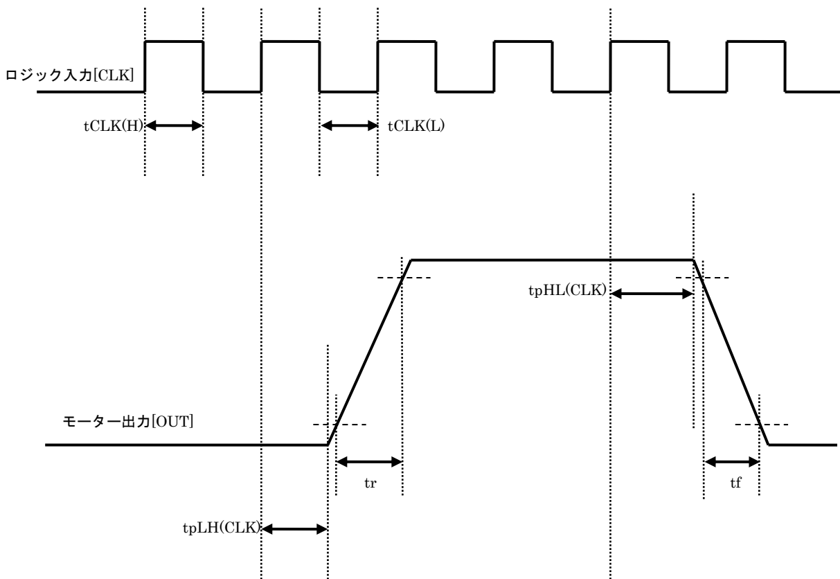
図 10.1 TB67S279FTG(CLK と出力の関係)
