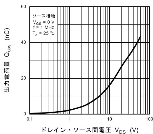
図 8.12 Q_{oss} - V_{DS}
