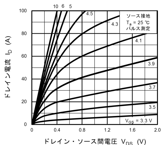
図 8.2 I_D - V_{DS}
