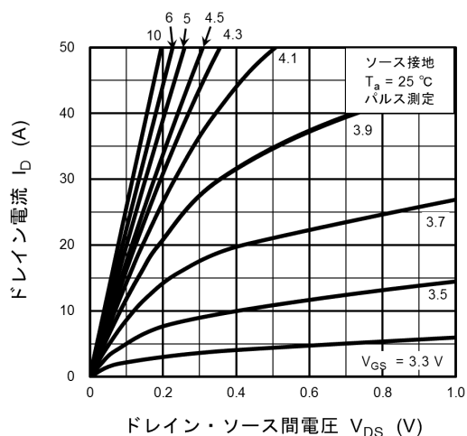
図 8.1 I_D - V_{DS}
