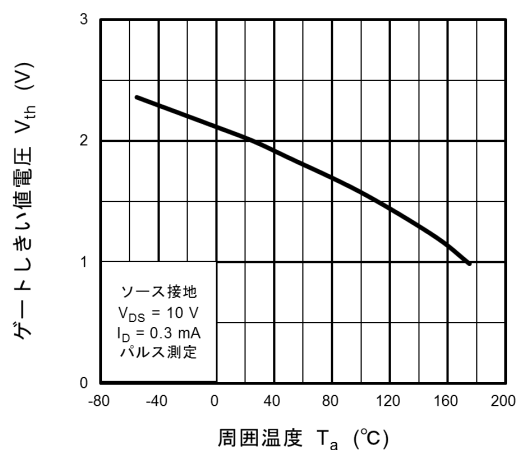
図 8.8 V_{th} - T_a
