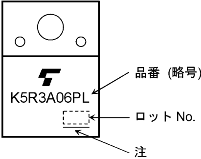
図 7.1 現品表示
