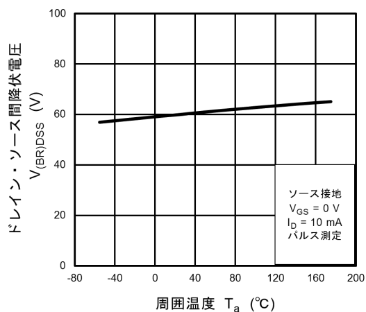
図 8.7 V_{(BR)DSS} - T_a
