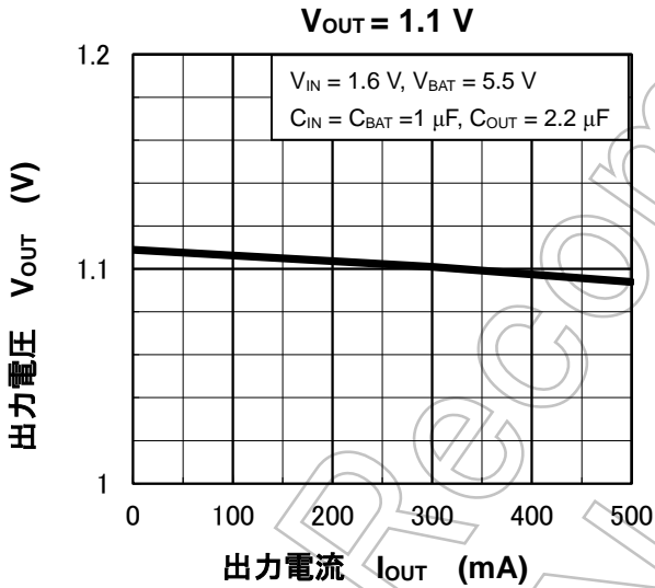
出力電圧—出力電流特性例
