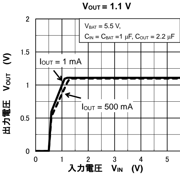
出力電圧—入力電圧特性例
