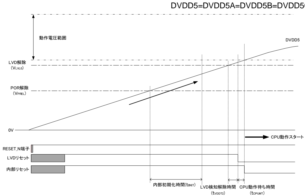
図 2.4 LVDリセットによるリセット動作
