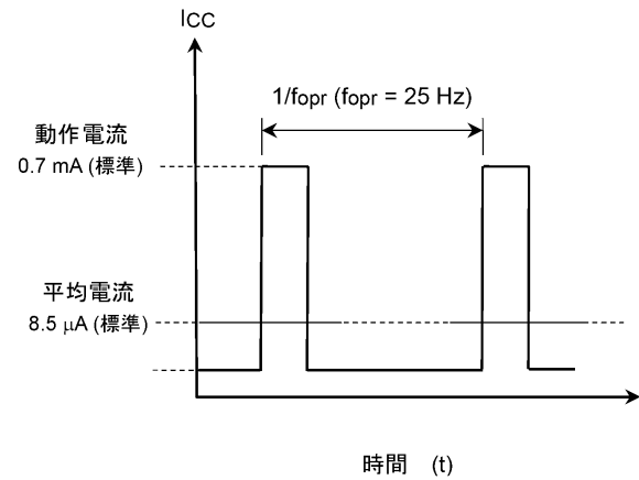
図 8.1.1 間欠動作時の消費電流
