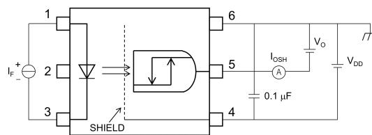
図 12.1.6 IOSH測定回路
