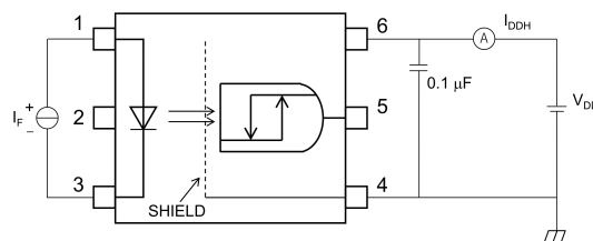
図 12.1.4 IDD_H測定回路
