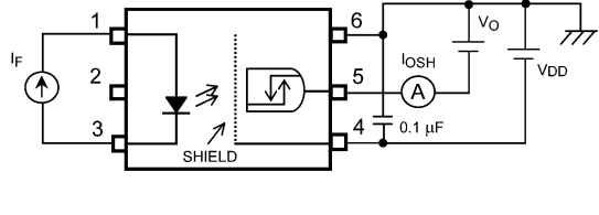
図 12.1.6 IOSH測定回路
