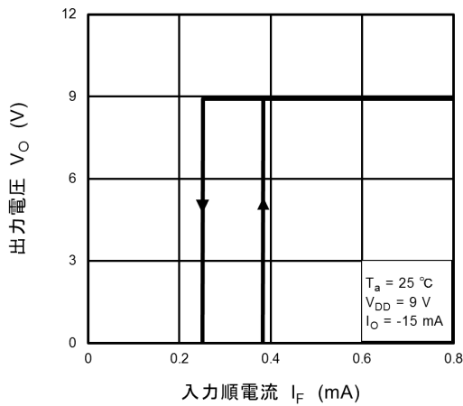
図 12.2.3 V_O - I_F(I_{HYS})
