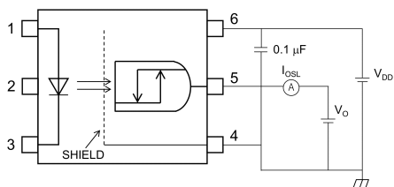
図 12.1.5 IOSL測定回路
