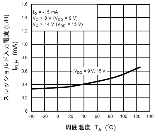
図 12.2.2 I_{FLH} - T_a
