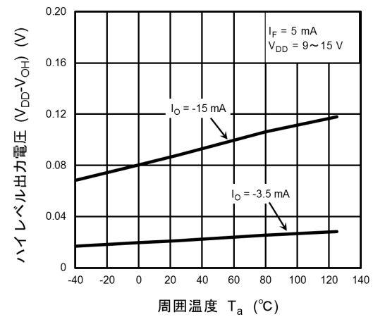
図 12.2.6 (V_{DD} - V_{OH}) - T_a
