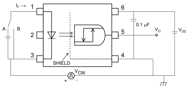
図 12.1.8 コモンモード過渡耐性測定回路, 波形
