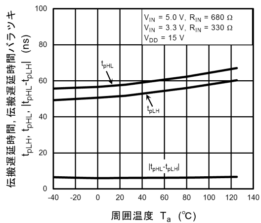
図 12.2.13 t_{pLH} , t_{pHL} , |t_{pHL}-t_{pLH}| - T_a
