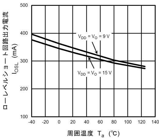
図 12.2.9 I_{OL} - T_a
