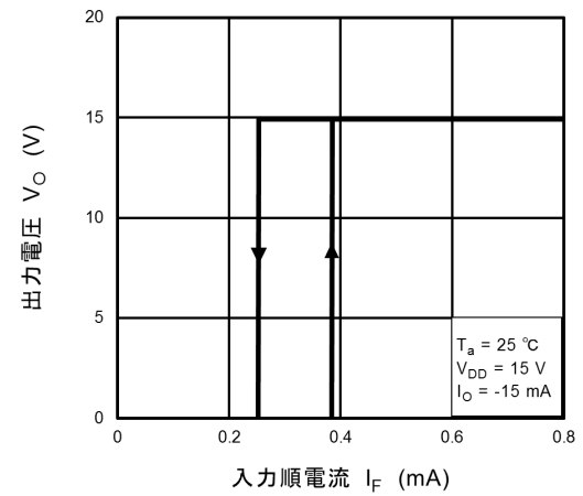
図 12.2.4 V_O - I_F(I_{HYS})
