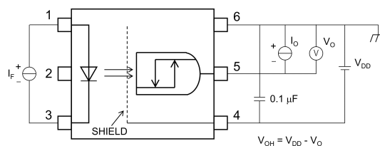
図 12.1.2 VOH測定回路
