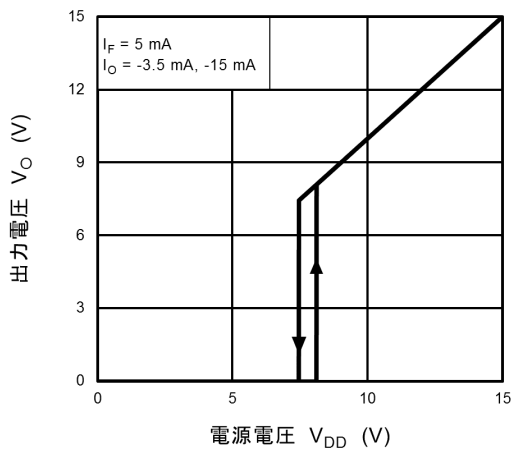
図 12.2.11 V_O - V_{DD}
