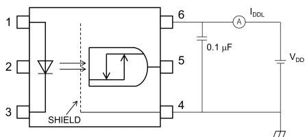
図 12.1.3 IDD_L測定回路
