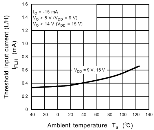
Fig. 12.2.2 I_{FLH} - T_a
