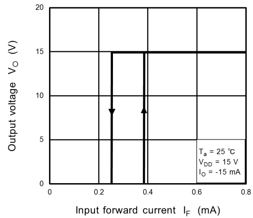
Fig. 12.2.4 V_O - I_F(I_{HYS})
