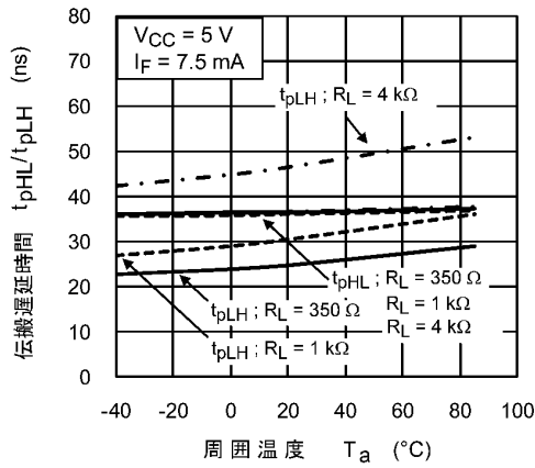
図 13.2.7 t_{pHL} / t_{pLH} - T_a
