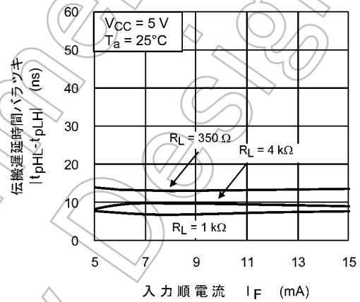
図 13.2.10 |t_{pHL} - t_{pLH}| - I_F
