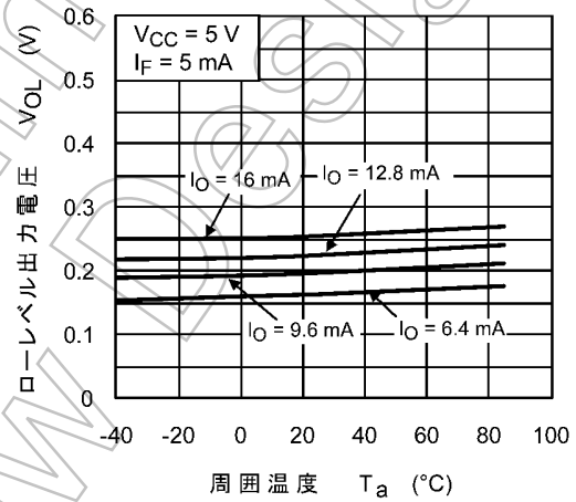
図 13.2.4 V_{OL} - T_a
