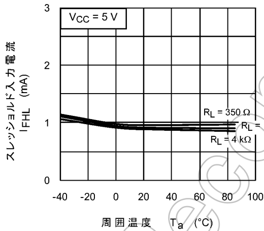
図 13.2.3 I_{FHL} - T_a
