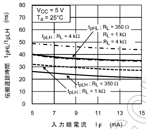
図 13.2.9 t_{pHL} / t_{pLH} - I_F
