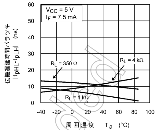
図 13.2.8 |t_{pHL} - t_{pLH}| - T_a
