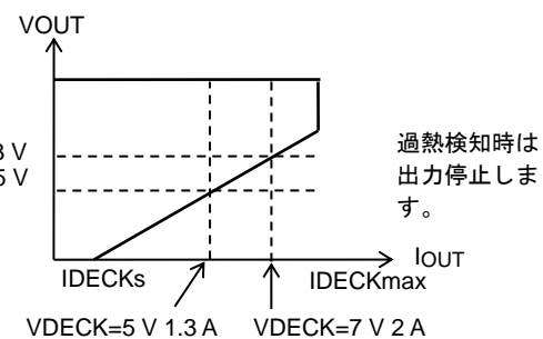
DECK 7.0 V/5.0 V 設定時負荷特性
