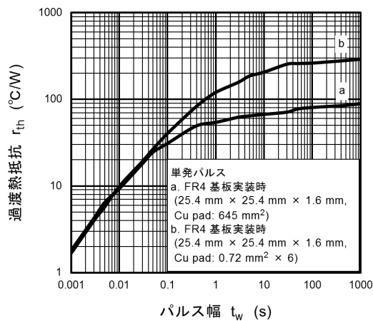
図 7.11 r_{th} - t_w
