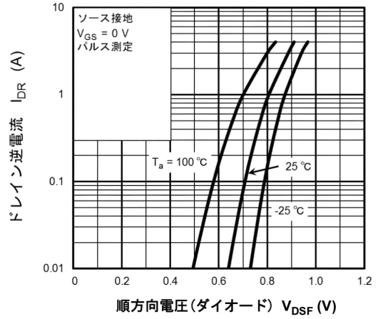
図 8.8 I DR - V DSF
