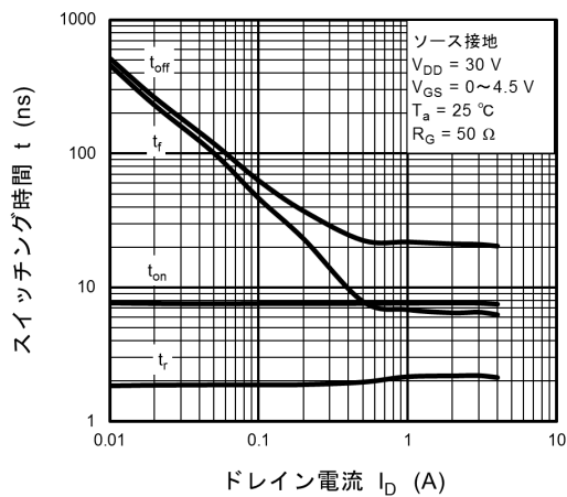
図 7.9 t - I_D
