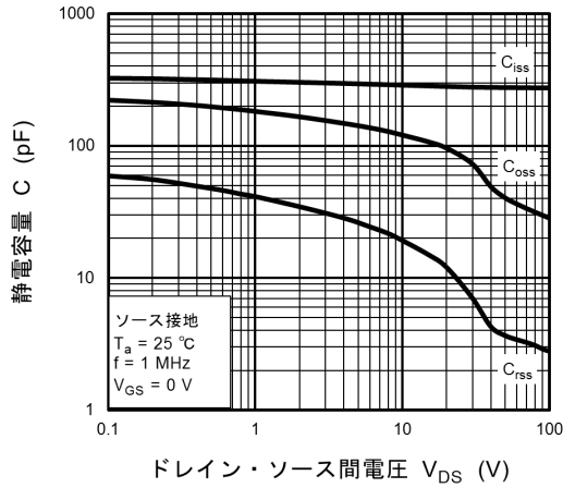
図 7.7 C - V_{DS}
