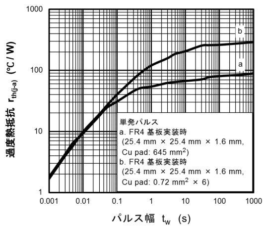
図 8.11 r th(j-a) - t w
