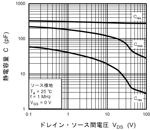
図 8.7 C - V DS
