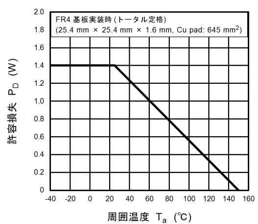
図 8.12 P_D - T_a
