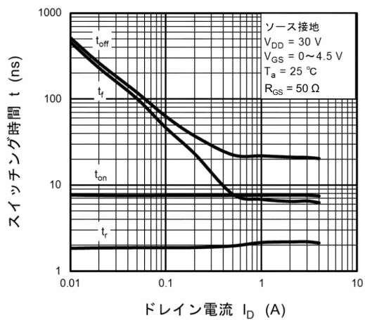
図 8.9 t - I_D
