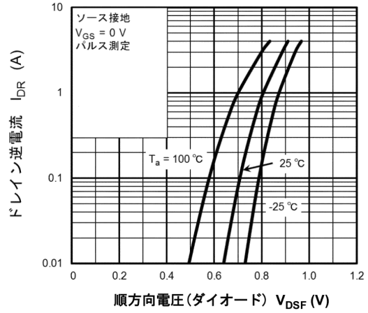
図 8.8 I_{DR} - V_{DSF}
