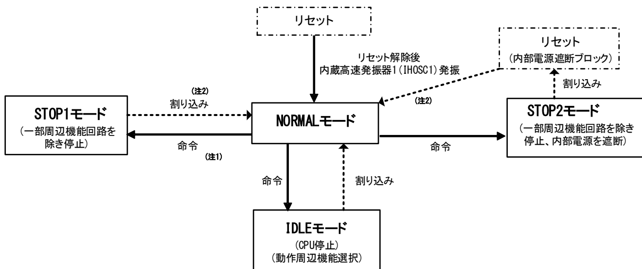
図 3.1 モード状態遷移
