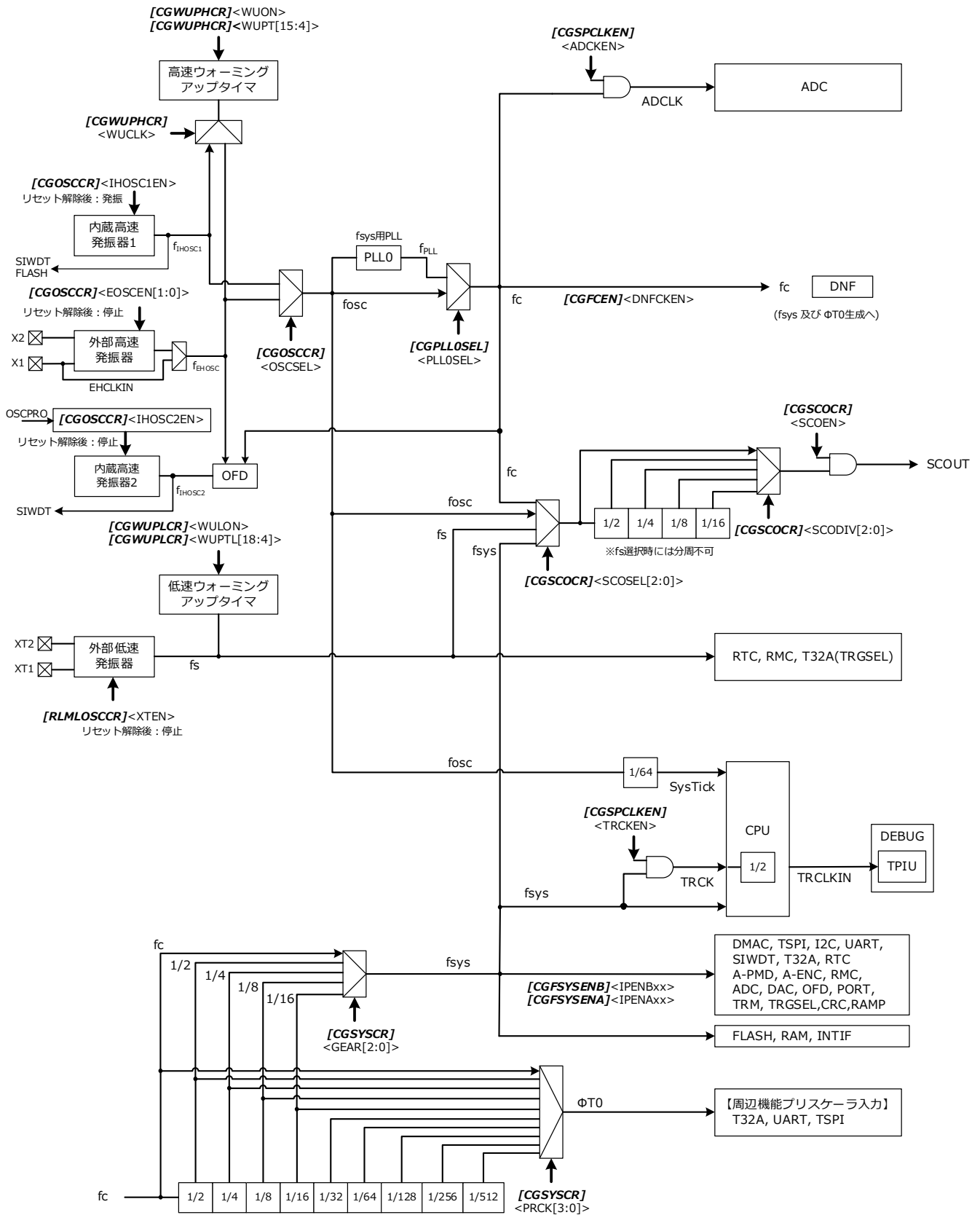
図 2.1 クロック系統図
