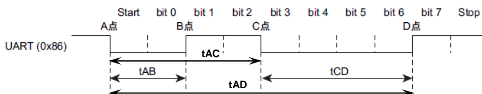
図 6.13 シリアル動作モード判定データ
