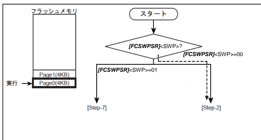
図 6.30 ユーザーブートプログラムの書き替え(1)
