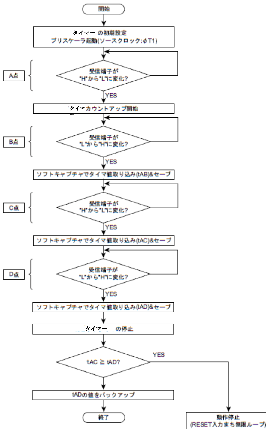
図 6.14 シリアル動作モード受信フローチャート
