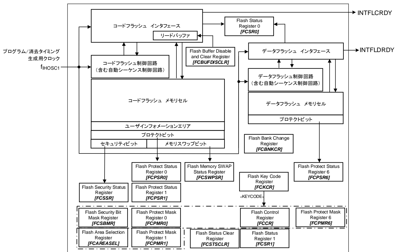
図 2.1 フラッシュメモリーのブロック図
