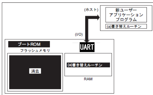
図 6.22 内蔵ブートプログラムを利用した書き替え手順(4)
