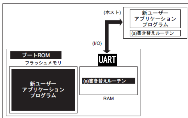
図 6.23 内蔵ブートプログラムを利用した書き替え手順(5)
