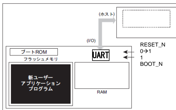
図 6.24 内蔵ブートプログラムを利用した書き替え手順(6)
