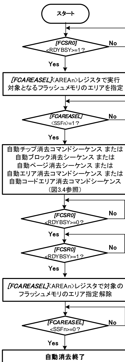
図 3.3 自動消去のフロー(1)
