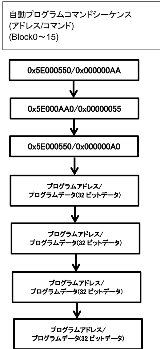
図 3.2 自動プログラムのフロー(2)
