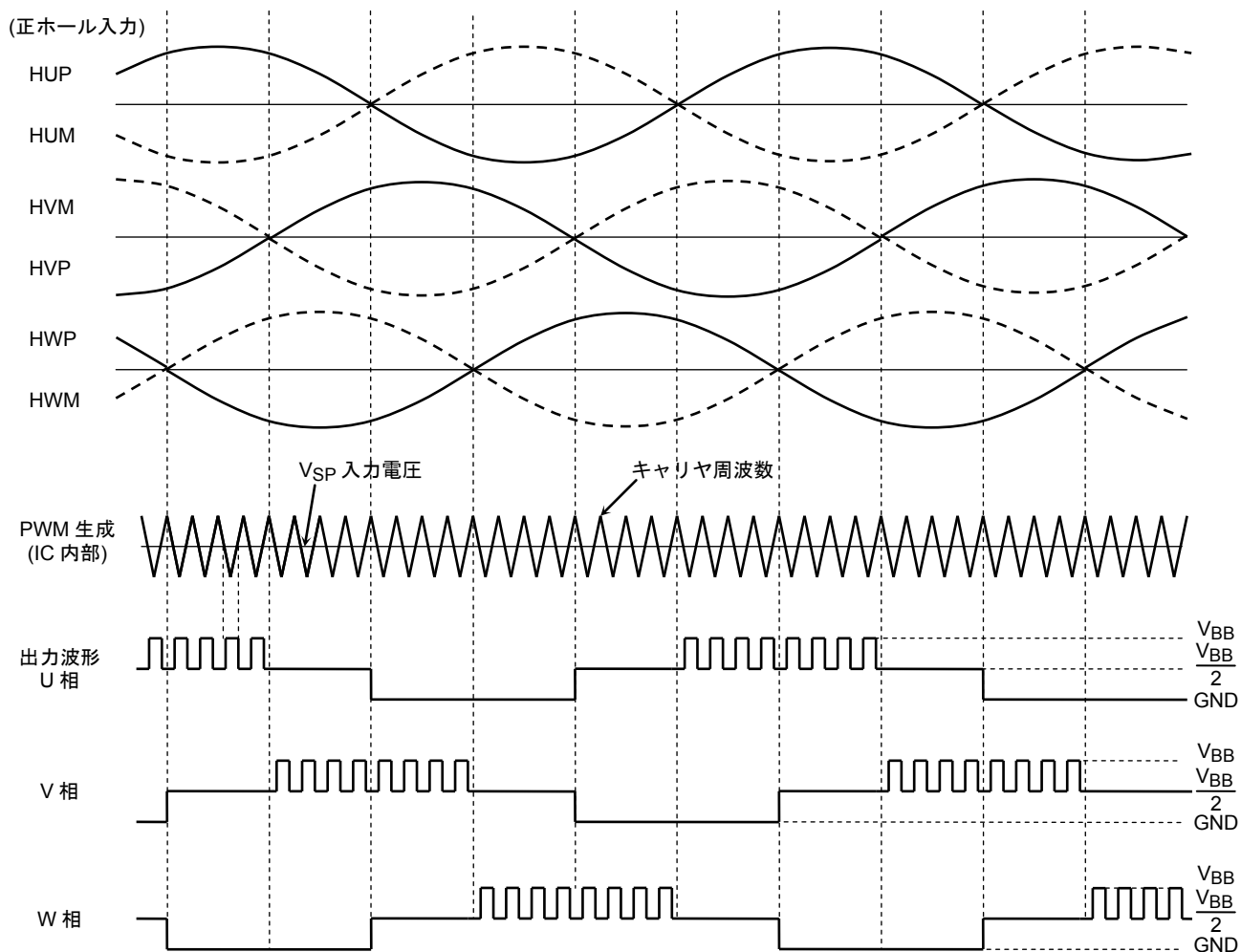
タイミングチャート 8 : 矩形波駆動の出力動作波形 (CW/CCW = L, LA = GND, 正ホール入力)
