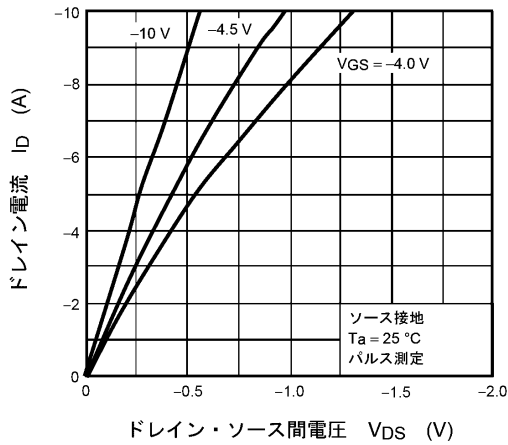
図 9.1 I_D - V_{DS}
