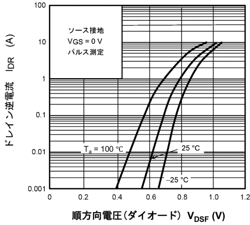
図 9.9 I_{DR} - V_{DSF}
