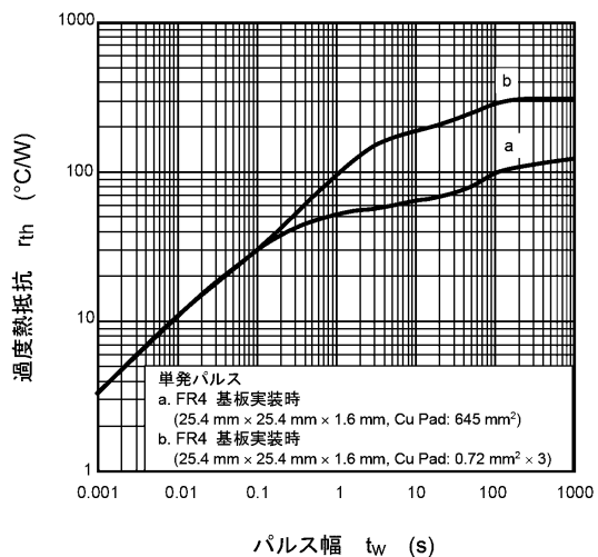
図 7.13 r_{th} - t_w
