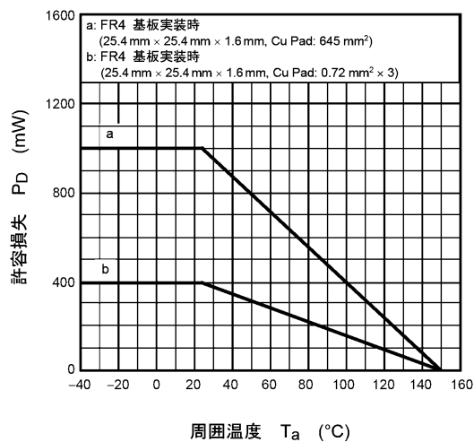
図 7.14 P_D - T_a
