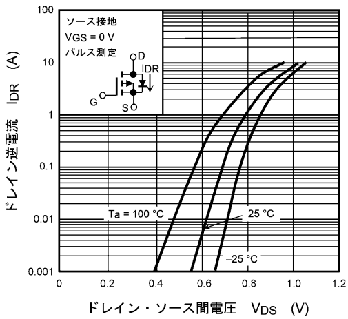
図 7.9 I_{DR} - V_{DS}
