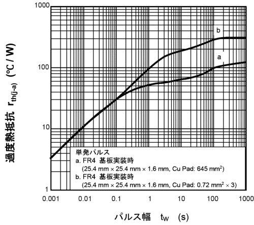
図 9.13 r_{th(j-a)} - t_w
