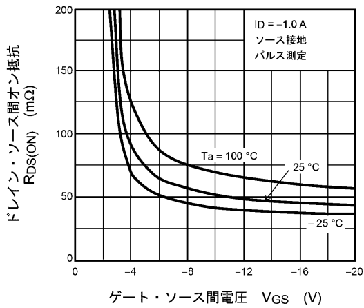
図 7.3 R_{DS(ON)} - V_{GS}
