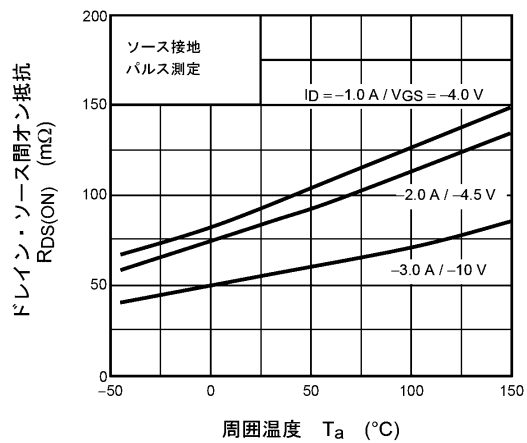
図 7.6 R_{DS(ON)} - T_a
