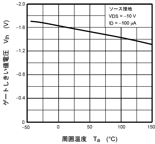
図 7.7 V_{th} - T_a
