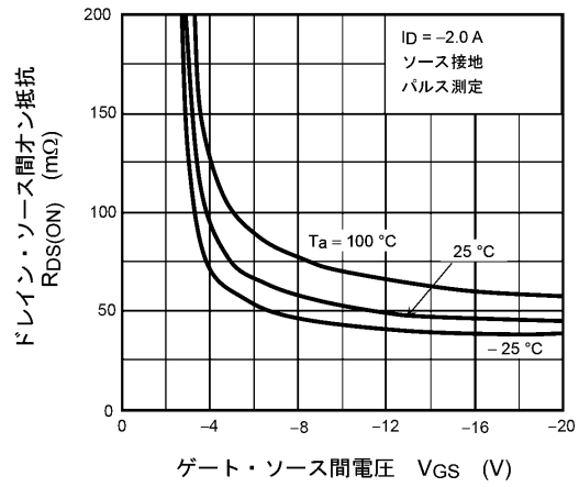
図 7.4 R_{DS(ON)} - V_{GS}
