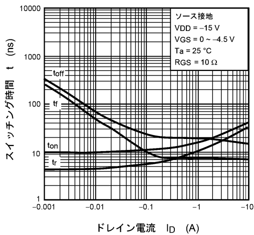
図 9.11 t - I_D
