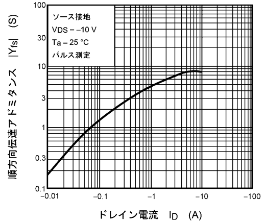
図 9.8 |Y_{fs}| - I_D
