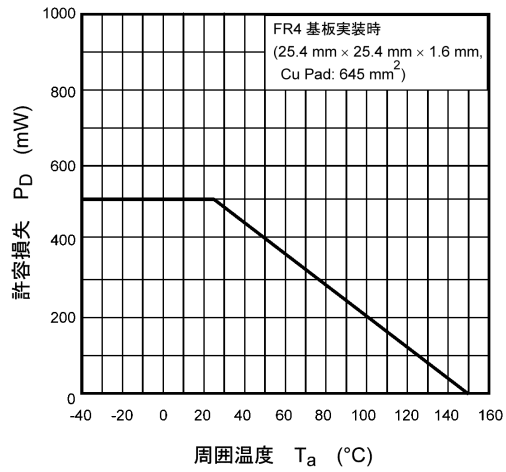
図 7.13 P_D - T_a
