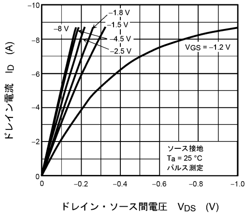
図 8.1 I_D - V_{DS}
