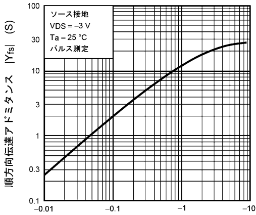
ドレイン電流 I_D (A) 図 8.7 |Y_{fs}| - I_D
