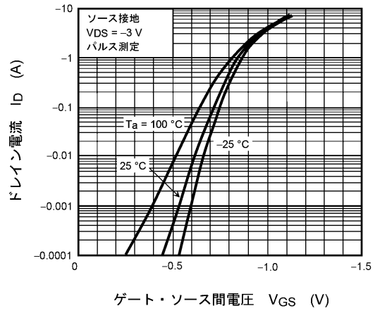
図 7.2 I_D - V_{GS}
