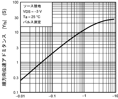
ドレイン電流 I_D (A) 図 7.7 |Y_{fs}| - I_D
