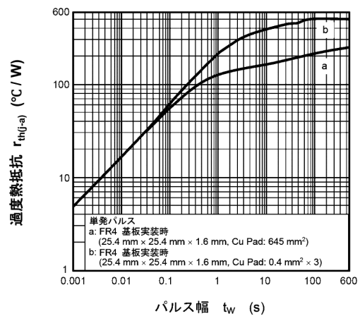
図 8.12 r_{th(j-a)} - t_w
