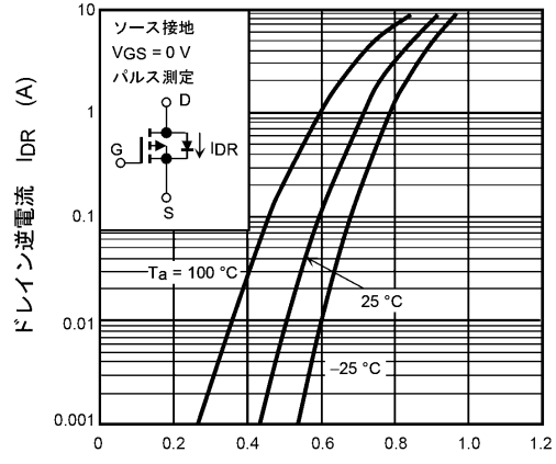
ドレイン・ソース間電圧 V_{DS} (V) 図 7.8 I_{DR} - V_{DS}
