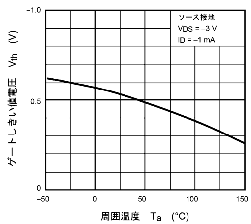
図 7.6 V_{th} - T_a
