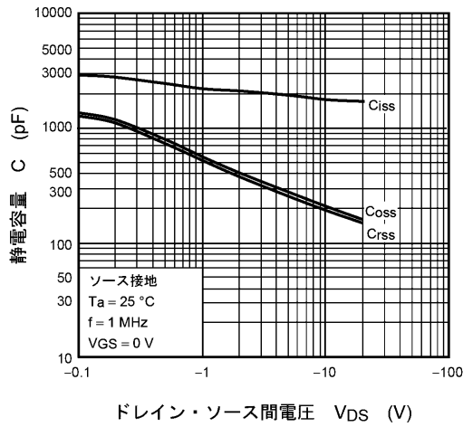
図 8.9 C - V_{DS}
