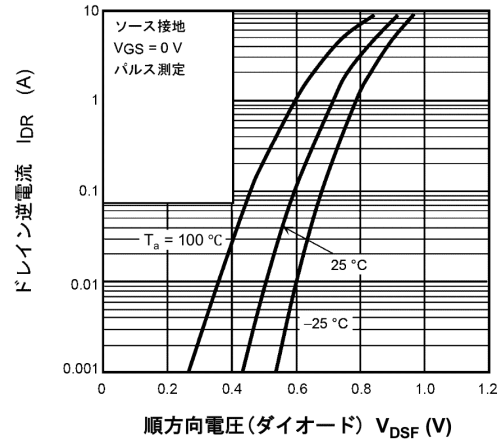
図 8.8 I_{DR} - V_{DSF}
