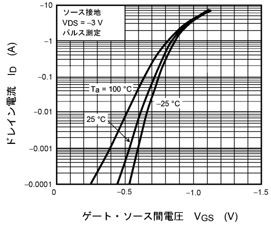
図 8.2 I_D - V_{GS}
