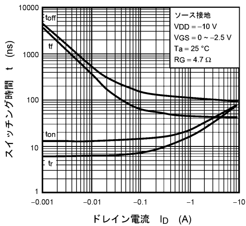
図 7.11 t - I_D
