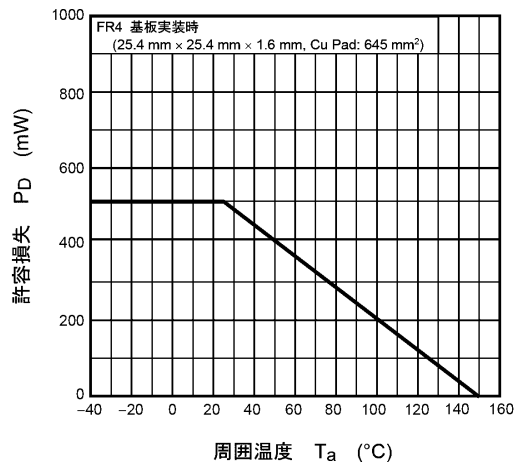
図 7.14 P_D - T_a
