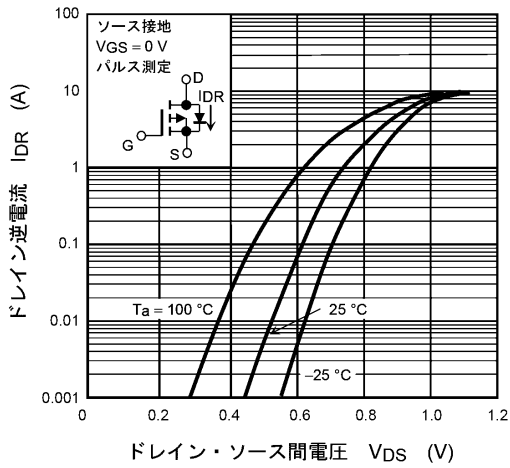
図 7.9 I_{DR} - V_{DS}
