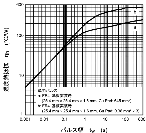
図 7.13 r_{th} - t_w
