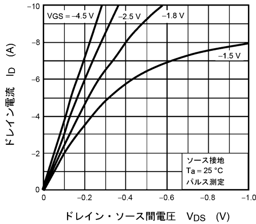
図 7.1 I_D - V_{DS}
