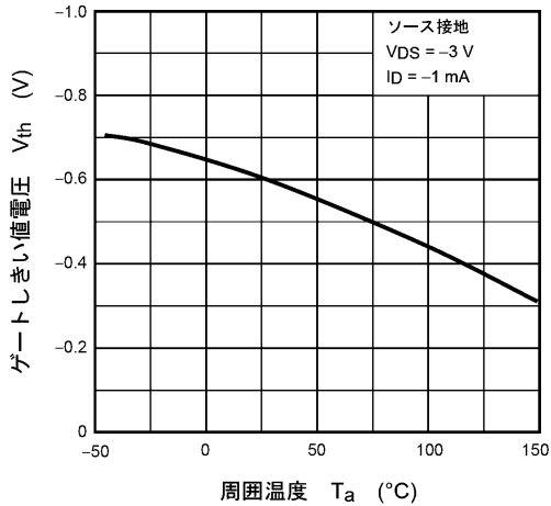
図 7.7 V_{th} - T_a
