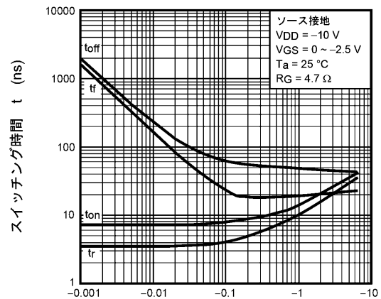
ドレイン電流 I_D (A) 図 8.10 t - I_D
