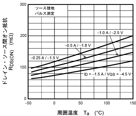
図 8.5 R_{DS(ON)} - T_a
