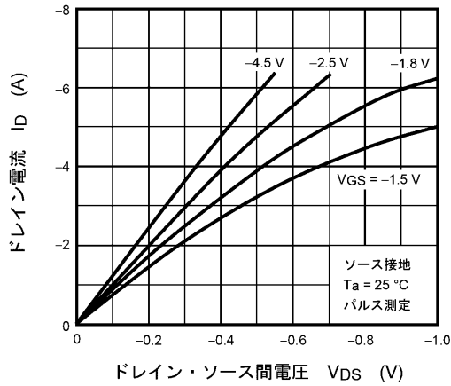
図 8.1 I_D - V_{DS}
