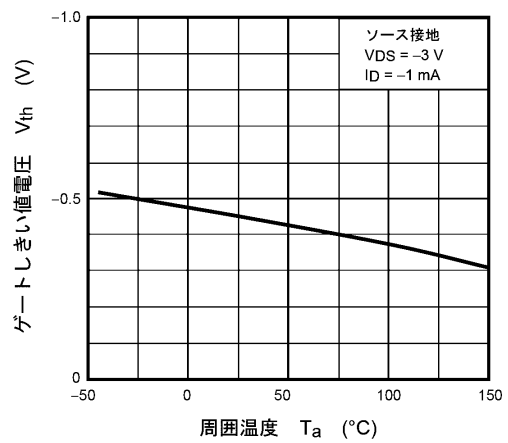
図 8.6 V_{th} - T_a
