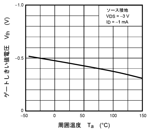
図 8.6 V_{th} - T_a
