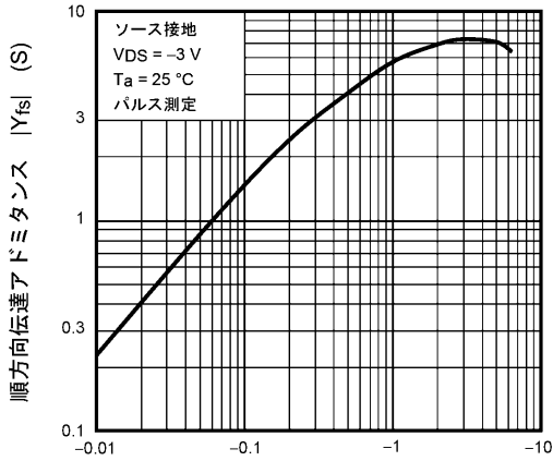
ドレイン電流 I_D (A) 図 8.7 |Y_{fs}| - I_D
