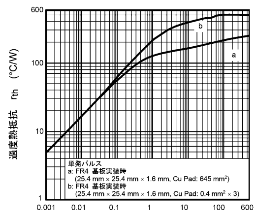
パルス幅 t_w (s) 図 8.12 r_{th} - t_w
