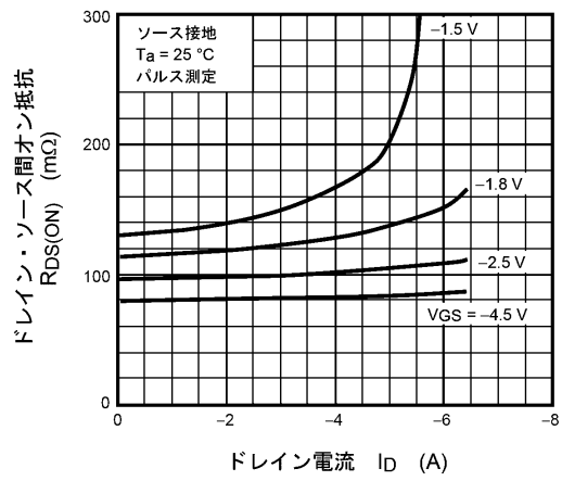
図 8.4 R_{DS(ON)} - I_D
