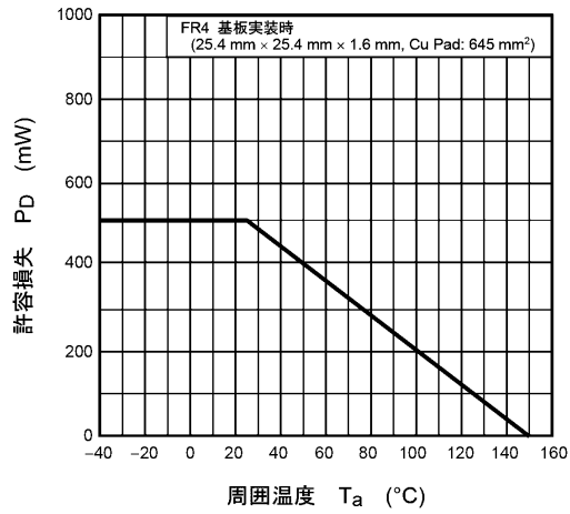
図 8.13 P_D - T_a
