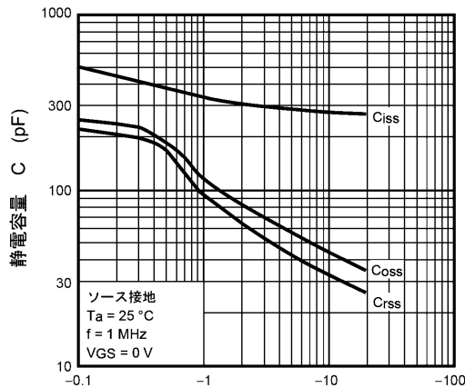
ドレイン・ソース間電圧 V_{DS} (V) 図 8.9 C - V_{DS}
