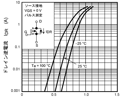
ドレイン・ソース間電圧 V_{DS} (V) 図 8.8 I_{DR} - V_{DS}
