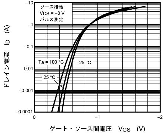
図 8.2 I_D - V_{GS}
