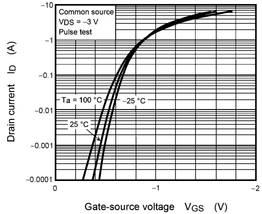
Fig. 8.2 I_D - V_{GS}
