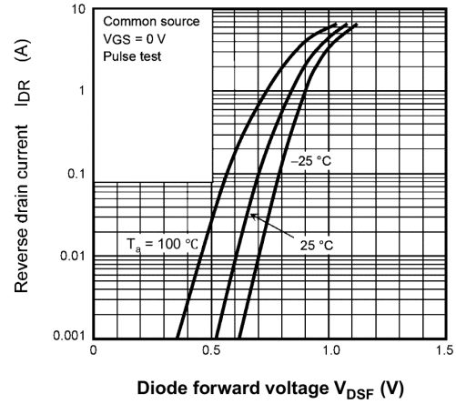
Fig. 8.8 I_{DR} - V_{DSF}
