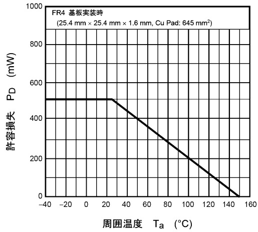
図 7.13 P_D - T_a
