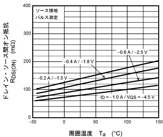
図 7.5 R_{DS(ON)} - T_a
