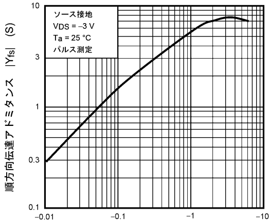
ドレイン電流 I_D (A) 図 7.7 |Y_{fs}| - I_D
