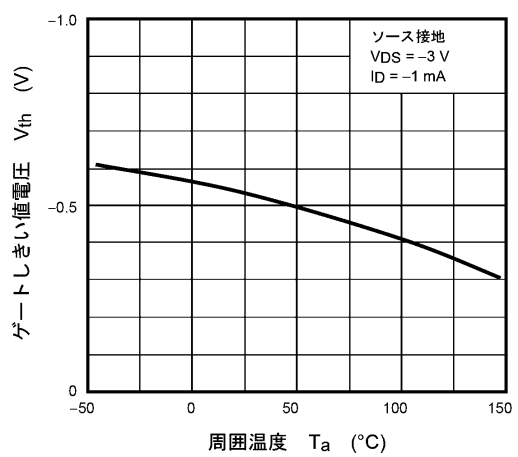
図 7.6 V_{th} - T_a
