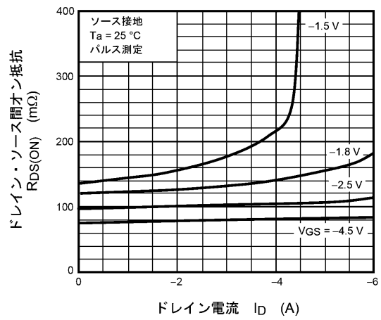
図 7.4 R_{DS(ON)} - I_D
