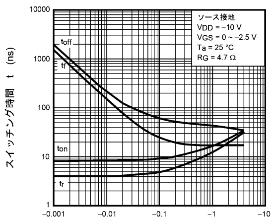
ドレイン電流 I_D (A) 図 7.10 t - I_D
