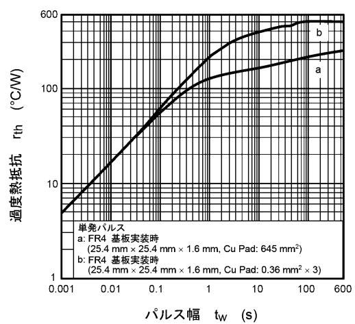
図 7.12 r_{th} - t_w
