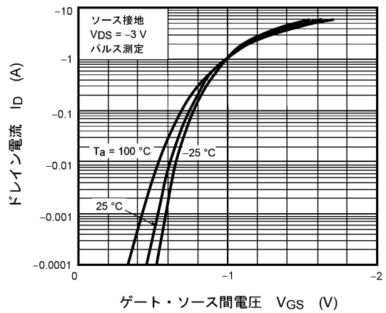
図 7.2 I_D - V_{GS}
