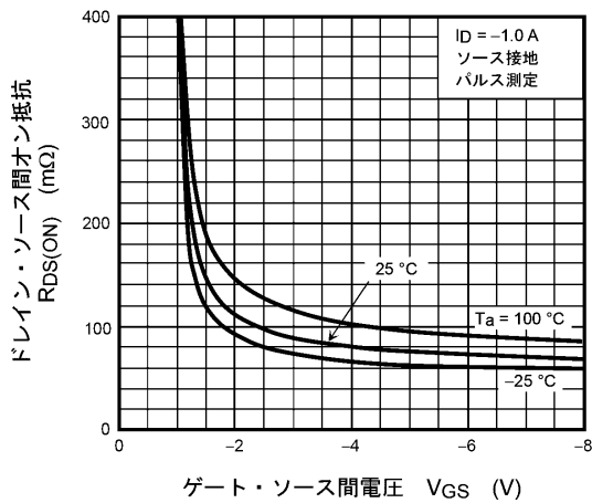
図 7.3 R_{DS(ON)} - V_{GS}
