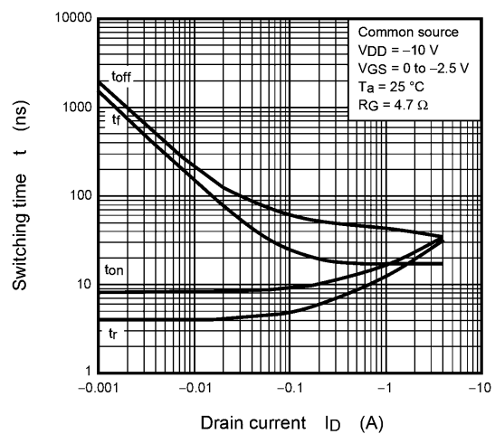
Fig. 7.10 t - I_D
