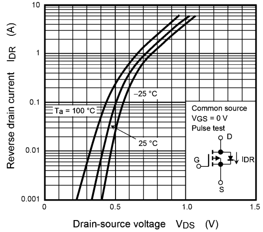
Fig. 8.8 I_{DR} - V_{DS}
