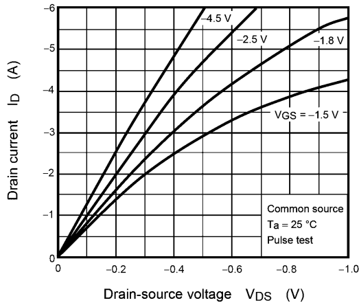
Fig. 7.1 I_D - V_{DS}
