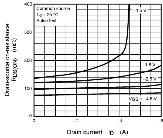
Fig. 7.4 R_{DS(ON)} - I_D
