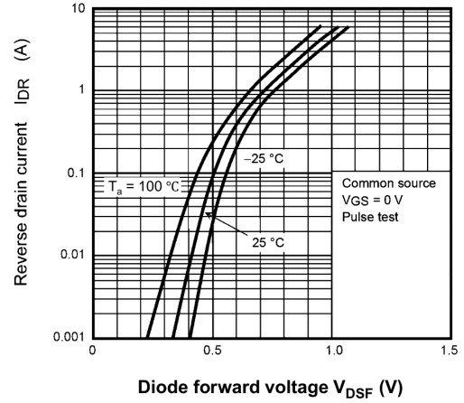
Fig. 8.8 I_{DR} - V_{DSF}
