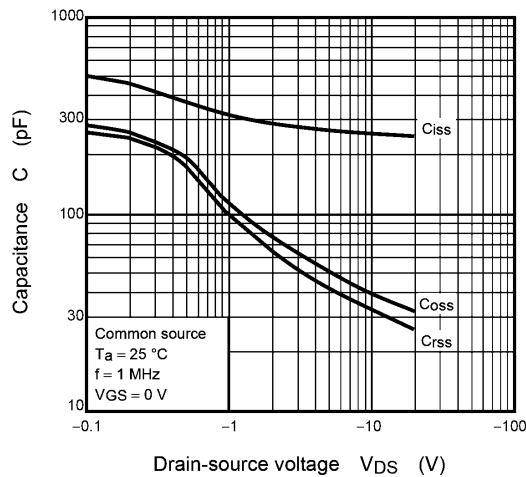
Fig. 7.9 C - V_{DS}
