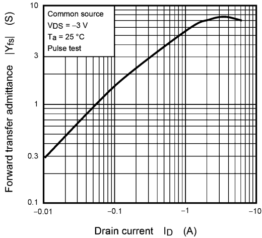
Fig. 8.7 |Y_{fs}| - I_D
