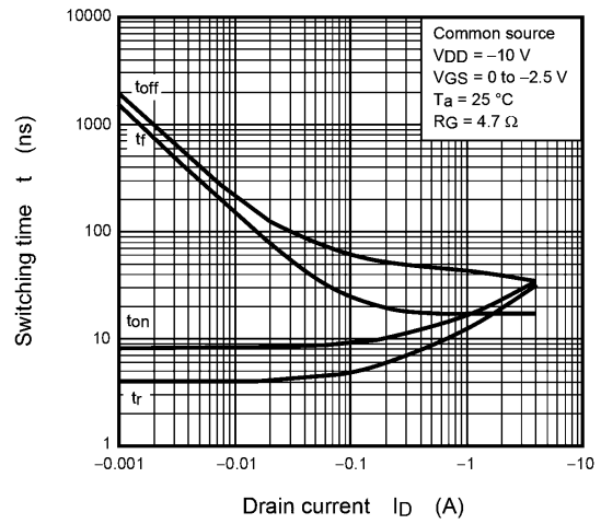
Fig. 8.10 t - I_D
