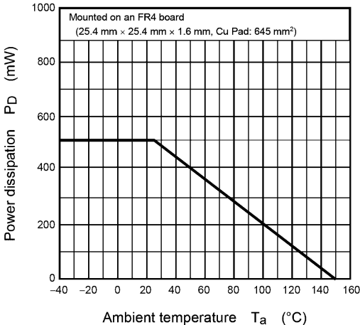
Fig. 7.13 P_D - T_a
