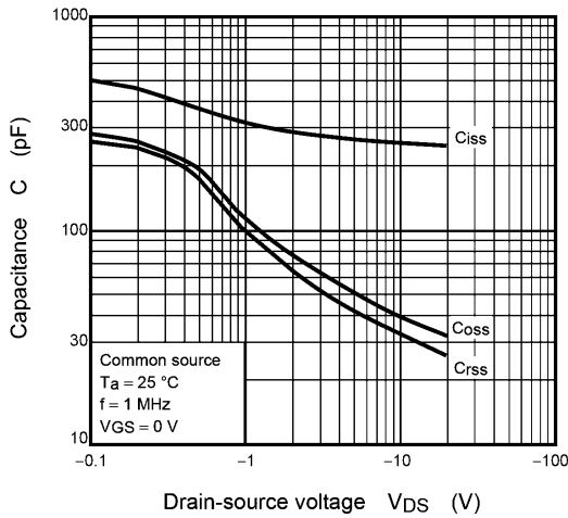
Fig. 8.9 C - V_{DS}
