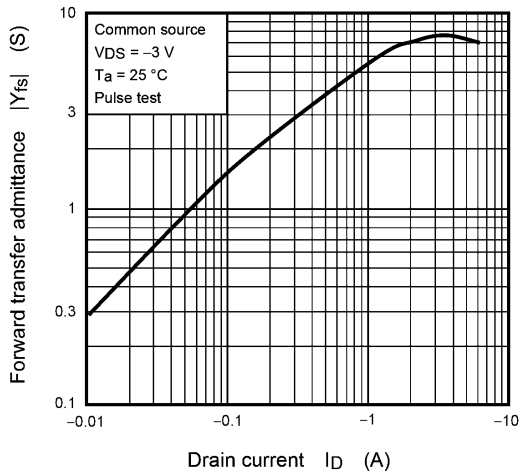
Fig. 7.7 |Y_{fs}| - I_D
