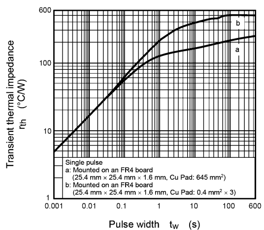
Fig. 8.12 r_{th} - t_w
