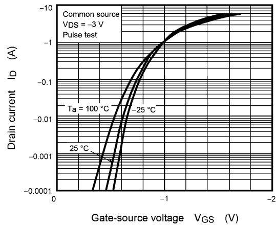
Fig. 7.2 I_D - V_{GS}
