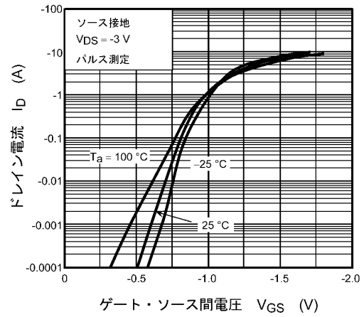
図 9.2 I_D - V_{GS}
