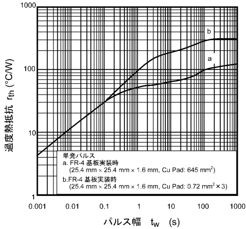
図 8.13 r_{th} - t_w
