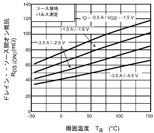
図 9.6 R_{DS(ON)} - T_a
