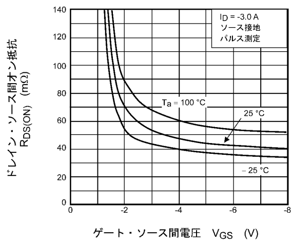
図 9.4 R_{DS(ON)} - V_{GS}
