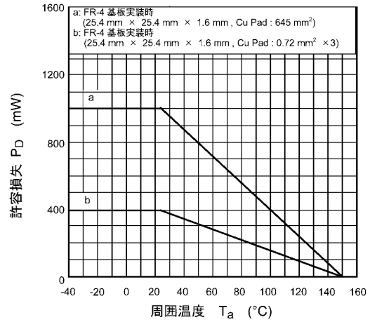
図 8.14 P_D - T_a
