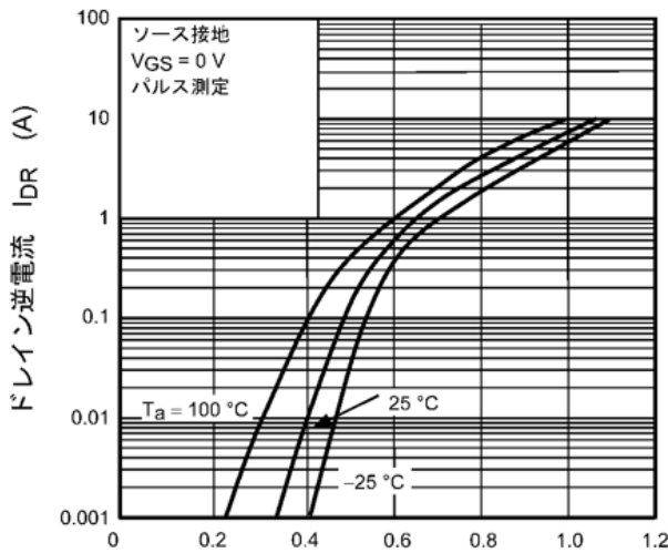
図 9.9 I_{DR} - V_{DS}
