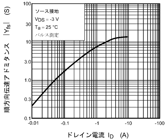
図 9.8 |Y_{fs}| - I_D
