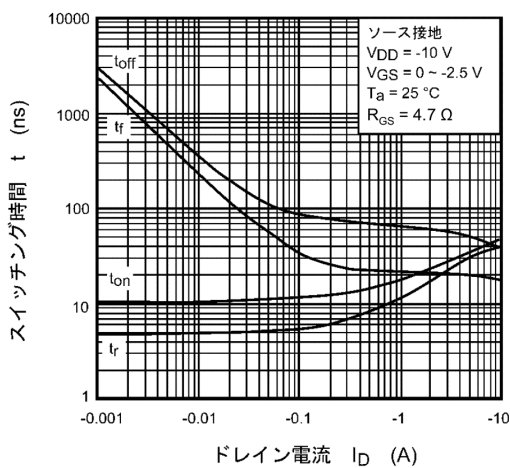
図 9.11 t - I_D
