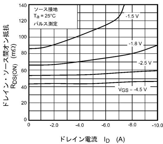
図 9.5 R_{DS(ON)} - I_D
