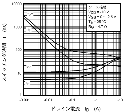
図 8.11 t - I_D
