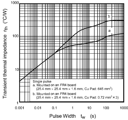
図 9.13 r_{th} - t_w
