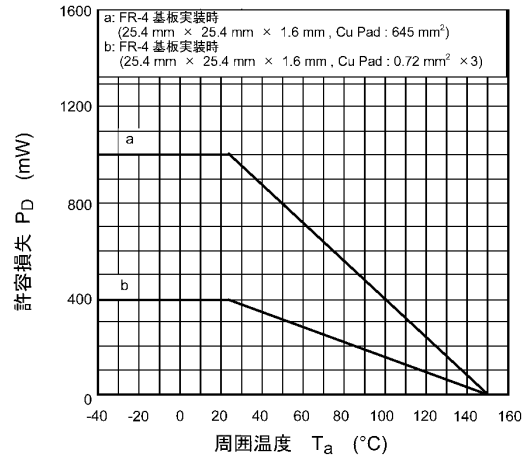
図 9.14 P_D - T_a
