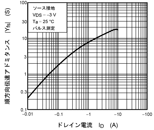
図 7.8 |Y_{fs}| - I_D
