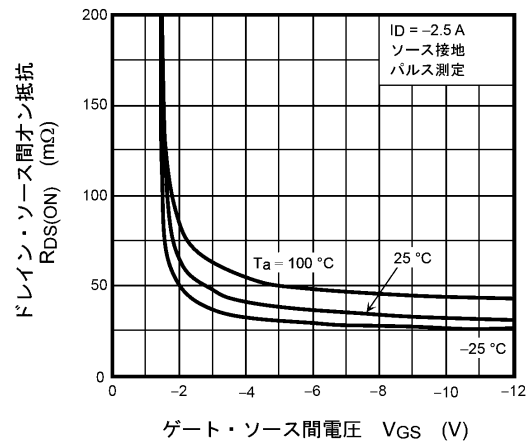
図 7.4 R_{DS(ON)} - V_{GS}
