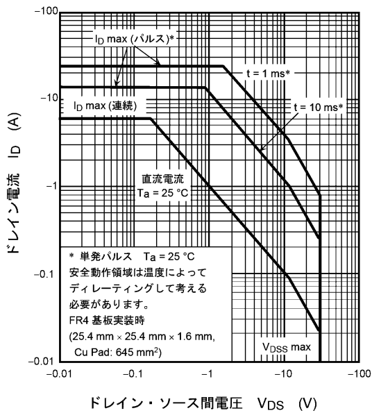
図 7.15 安全動作領域
