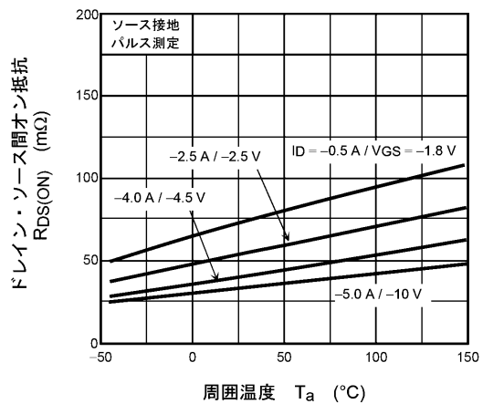
図 8.6 R_{DS(ON)} - T_a
