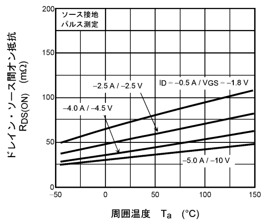
図 7.6 R_{DS(ON)} - T_a
