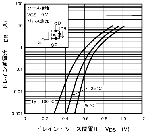
図 7.9 I_{DR} - V_{DS}
