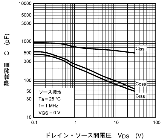
図 7.10 C - V_{DS}
