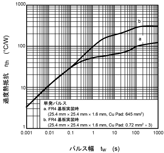
図 7.13 r_{th} - t_w
