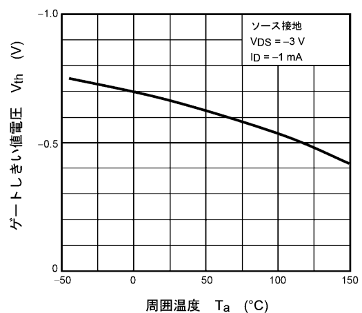
図 8.6 V_{th} - T_a
