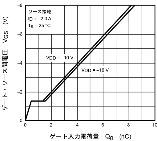
ゲート入力電荷量 Q_g (nC) 図 8.11 ダイナミック入力特性
