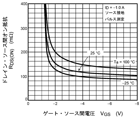
図 7.3 R_{DS(ON)} - V_{GS}
