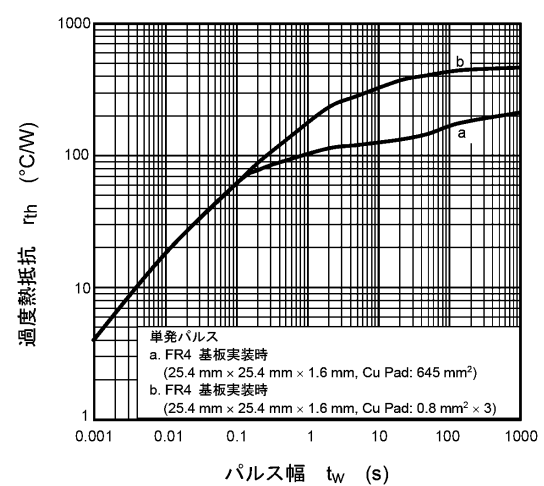
図 7.12 r_{th} - t_w
