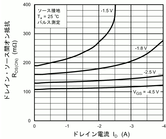
図 8.4 R_{DS(ON)} - I_D
