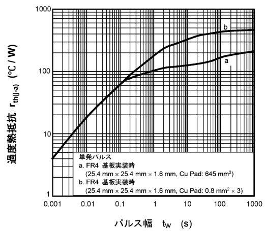
パルス幅 t_w (s) 図 8.12 r_{th(j-a)} - t_w
