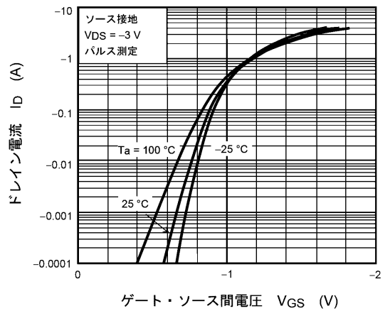
図 8.2 I_D - V_{GS}
