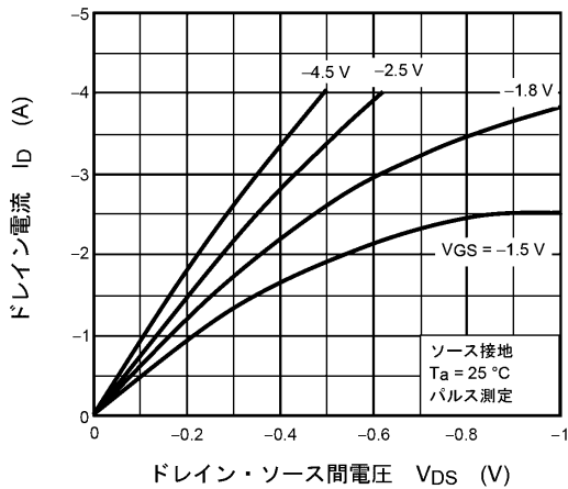
図 8.1 I_D - V_{DS}
