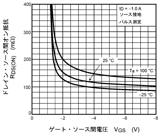
図 8.3 R_{DS(ON)} - V_{GS}
