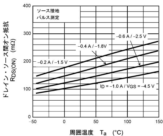
図 7.5 R_{DS(ON)} - T_a
