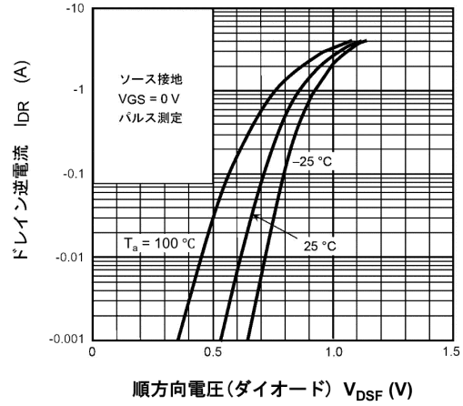
順方向電圧(ダイオード) V_{DSF} (V) 図 8.8 I_{DR} - V_{DSF}
