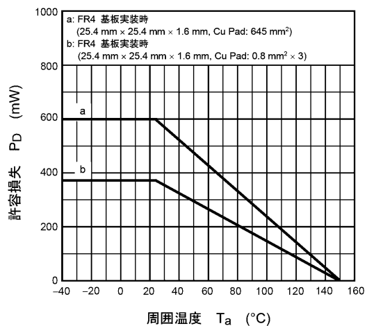
図 7.13 P_D - T_a
