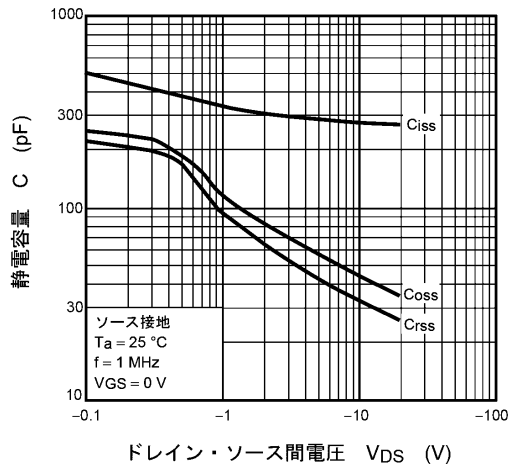
ドレイン・ソース間電圧 V_{DS} (V) 図 9.9 C - V_{DS}
