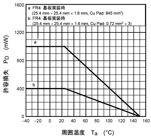
図 9.13 P_D - T_a
