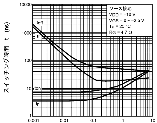
ドレイン電流 I_D (A) 図 8.10 t - I_D
