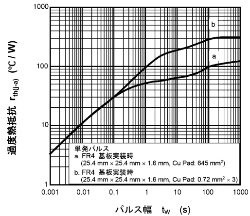
図 9.12 r_{th(j-a)} - t_w
