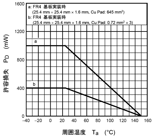
図 7.13 P_D - T_a
