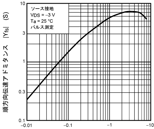
ドレイン電流 I_D (A) 図 9.7 |Y_{fs}| - I_D
