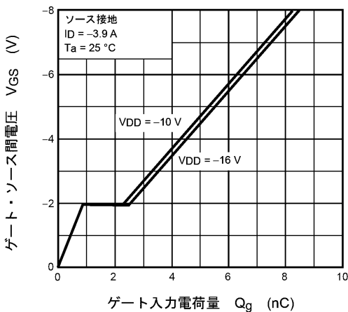
ゲート入力電荷量 Q_g (nC) 図 9.11 ダイナミック入力特性
