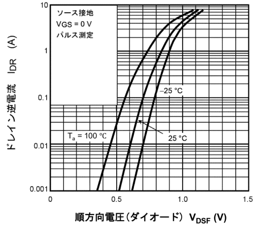
図 9.8 I_{DR} - V_{DSF}
