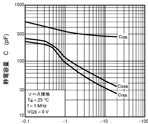
ドレイン・ソース間電圧 V_{DS} (V) 図 8.9 C - V_{DS}
