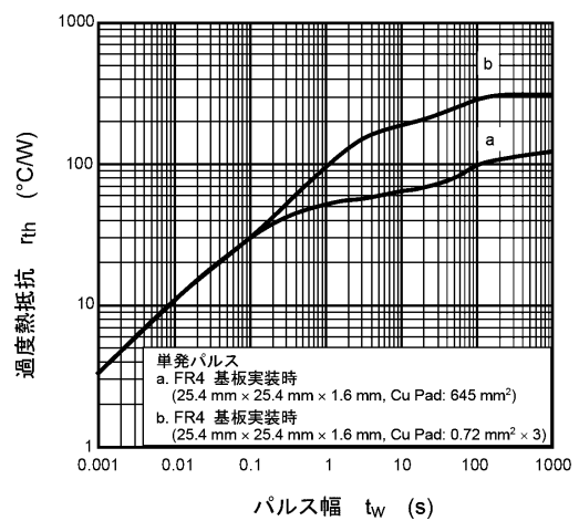
図 7.12 r_{th} - t_w
