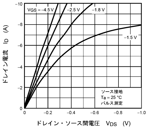
図 7.1 I_D - V_{DS}
