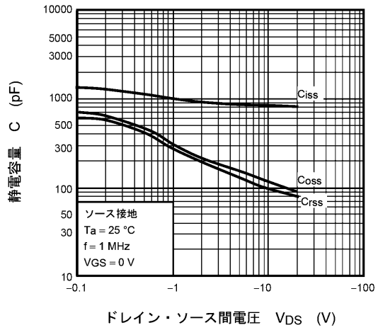
図 7.10 C - V_{DS}
