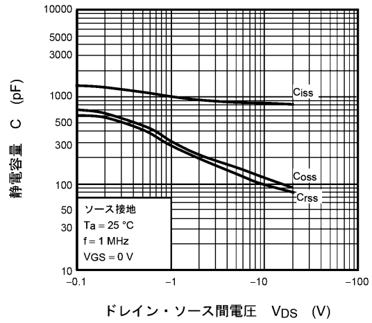
図 8.10 C - V_{DS}
