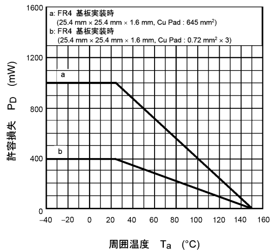
図 7.14 P_D - T_a
