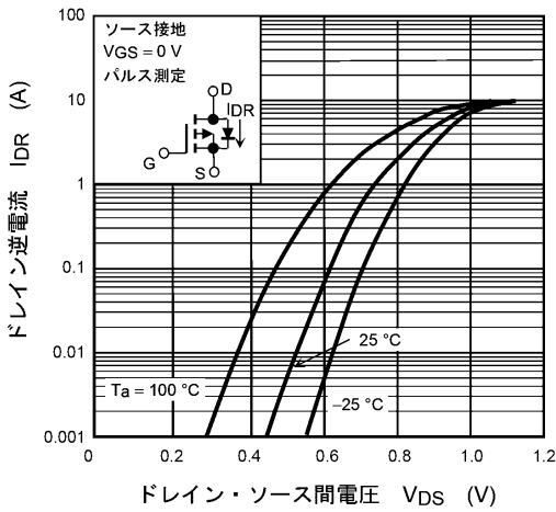
図 7.9 I_{DR} - V_{DS}
