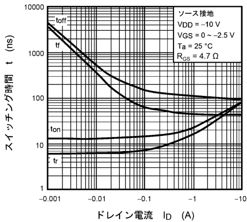
図 9.11 t - I_D
