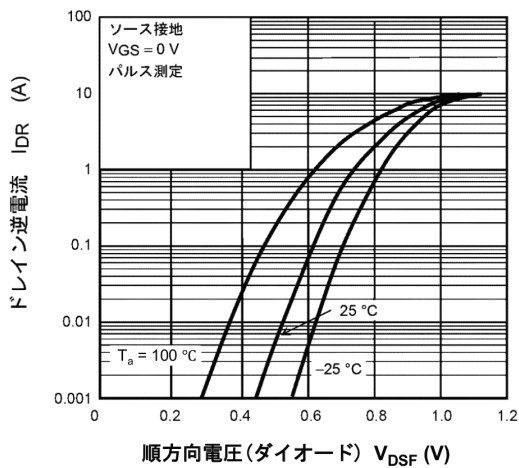
図 9.9 I_{DR} - V_{DSF}
