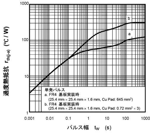
図 9.13 r_{th(j-a)} - t_w
