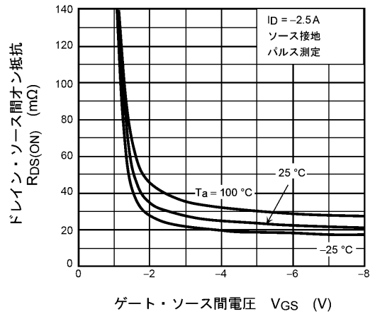
図 9.4 R_{DS(ON)} - V_{GS}
