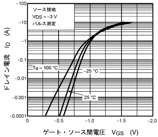
図 7.2 I_D - V_{GS}
