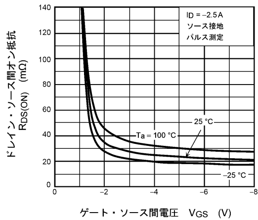
図 7.4 R_{DS(ON)} - V_{GS}
