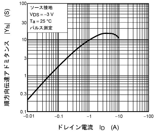
図 7.8 |Y_{fs}| - I_D
