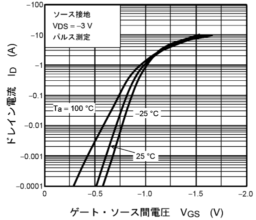
図 9.2 I_D - V_{GS}
