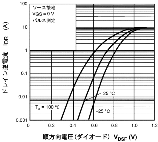
図 9.9 I_{DR} - V_{DSF}
