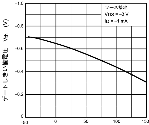
図 7.7 V_{th} - T_a
