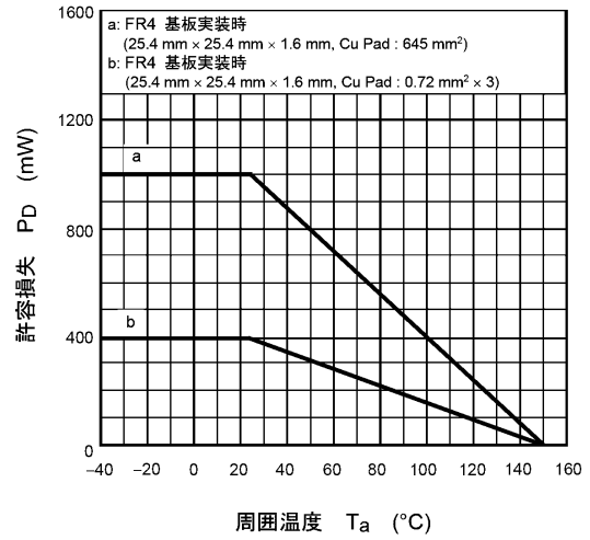
図 8.14 P_D - T_a
