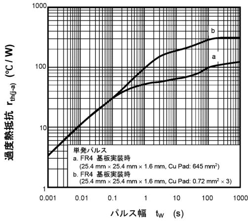
図 9.13 r_{th(j-a)} - t_w
