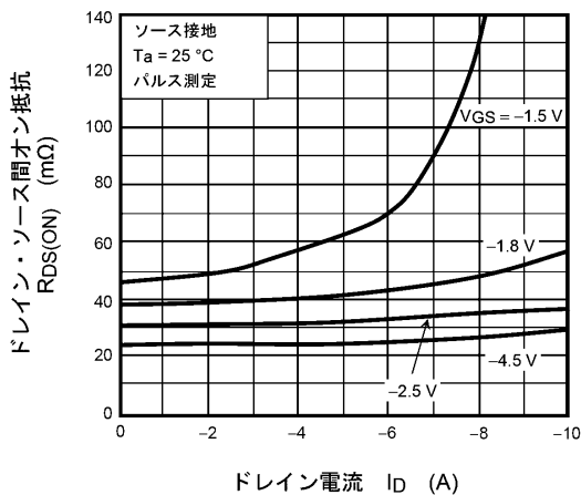
図 9.5 R_{DS(ON)} - I_D
