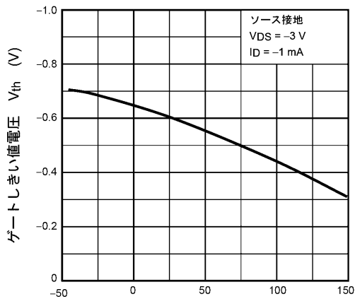
図 9.7 V_{th} - T_a
