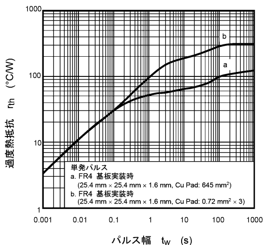
図 7.13 r_{th} - t_w
