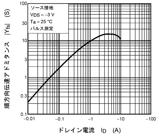
図 9.8 |Y_{fs}| - I_D
