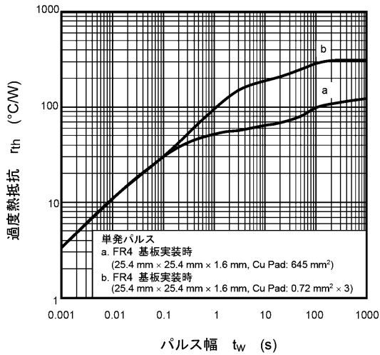
図 8.13 r_{th} - t_w
