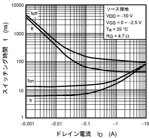
図 7.11 t - I_D
