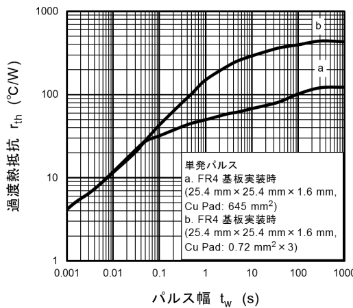
図 8.11 r_{th} - t_w
