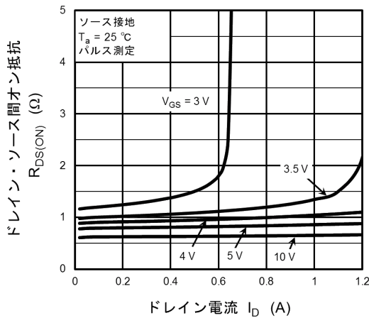
図 7.5 R_{DS(ON)} - I_D
