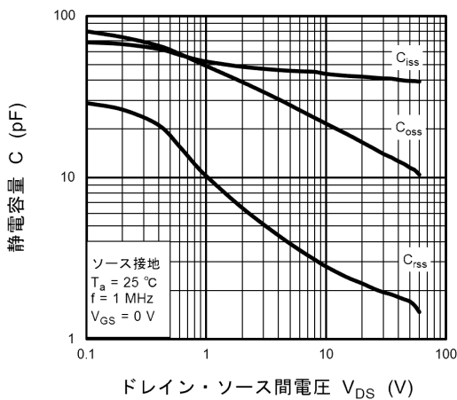
図 7.9 C - V_{DS}
