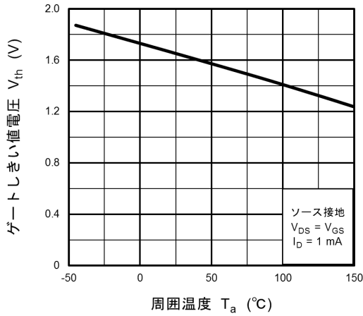
図 8.7 V_{th} - T_a
