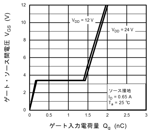
図 7.10 ダイナミック入力
