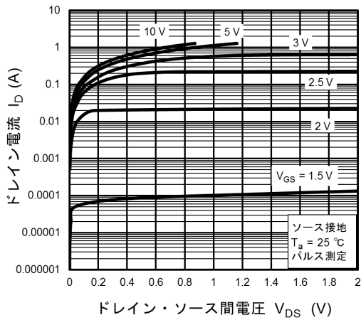
図 7.1 I_D - V_{DS}
