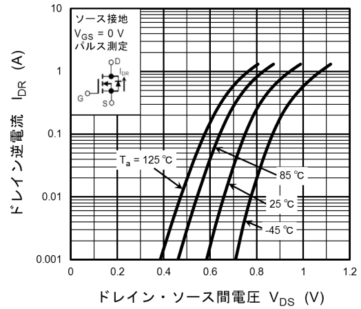
図 7.8 I_{DR} - V_{DS}
