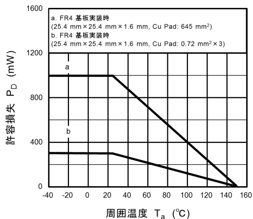
図 7.13 P_D - T_a
