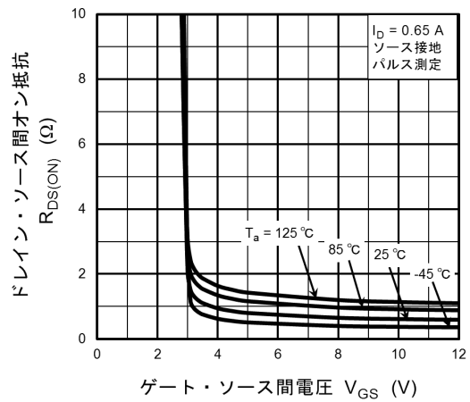
図 7.4 R_{DS(ON)} - V_{GS}
