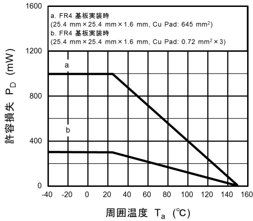
図 8.13 P_D - T_a
