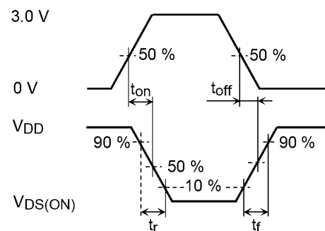
図 5.3.2 入力波形/出力波形
