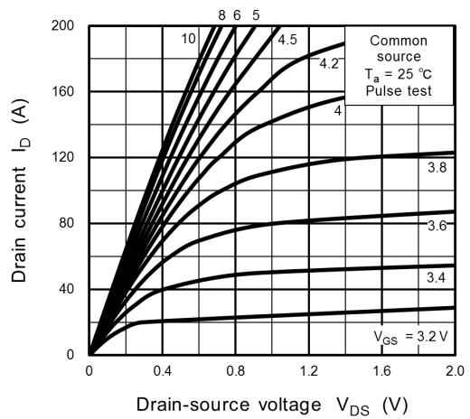
Fig. 8.2 I_D - V_{DS}
