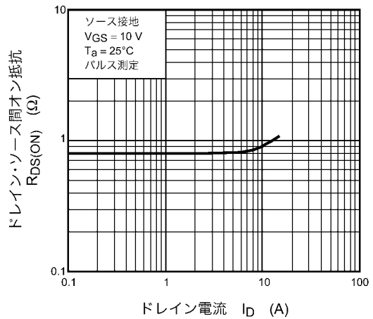
図 8.6 R_{DS(ON)} - I_D
