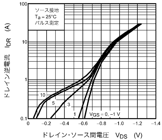
図 8.8 I_{DR} - V_{DS}
