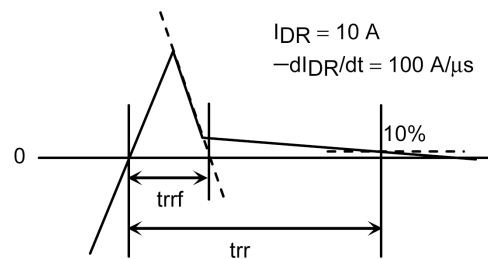
図 6.4.1 逆回復時間
