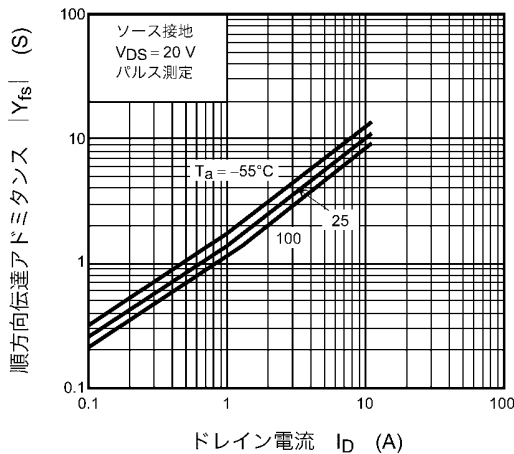
図 8.5 |Y_{fs}| - I_D
