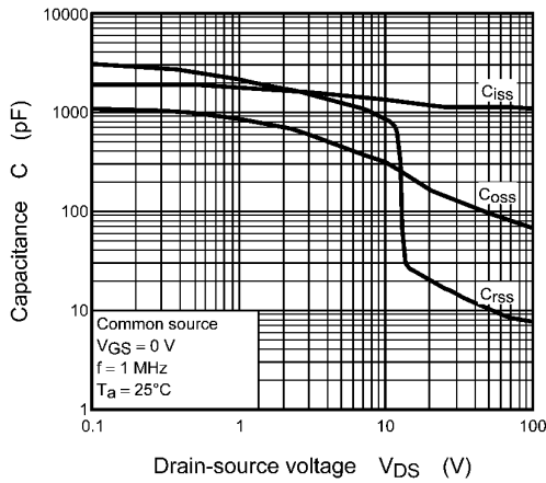
Fig. 8.9 C - V_{DS}
