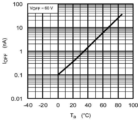
Fig. 12.9 I_{OFF} - T_a
